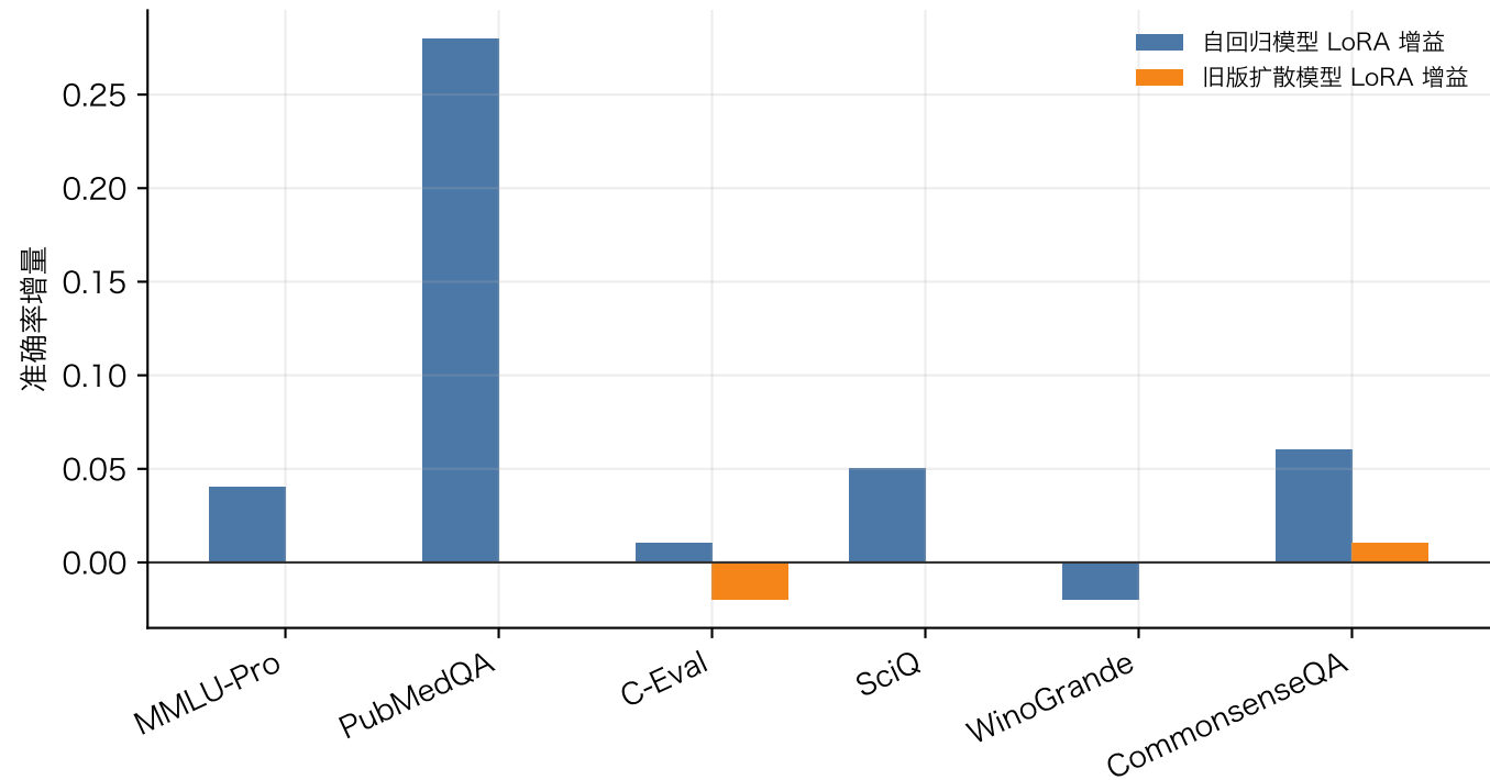
旧版 LoRA 审计：自回归模型更容易吸收固定标签监督
