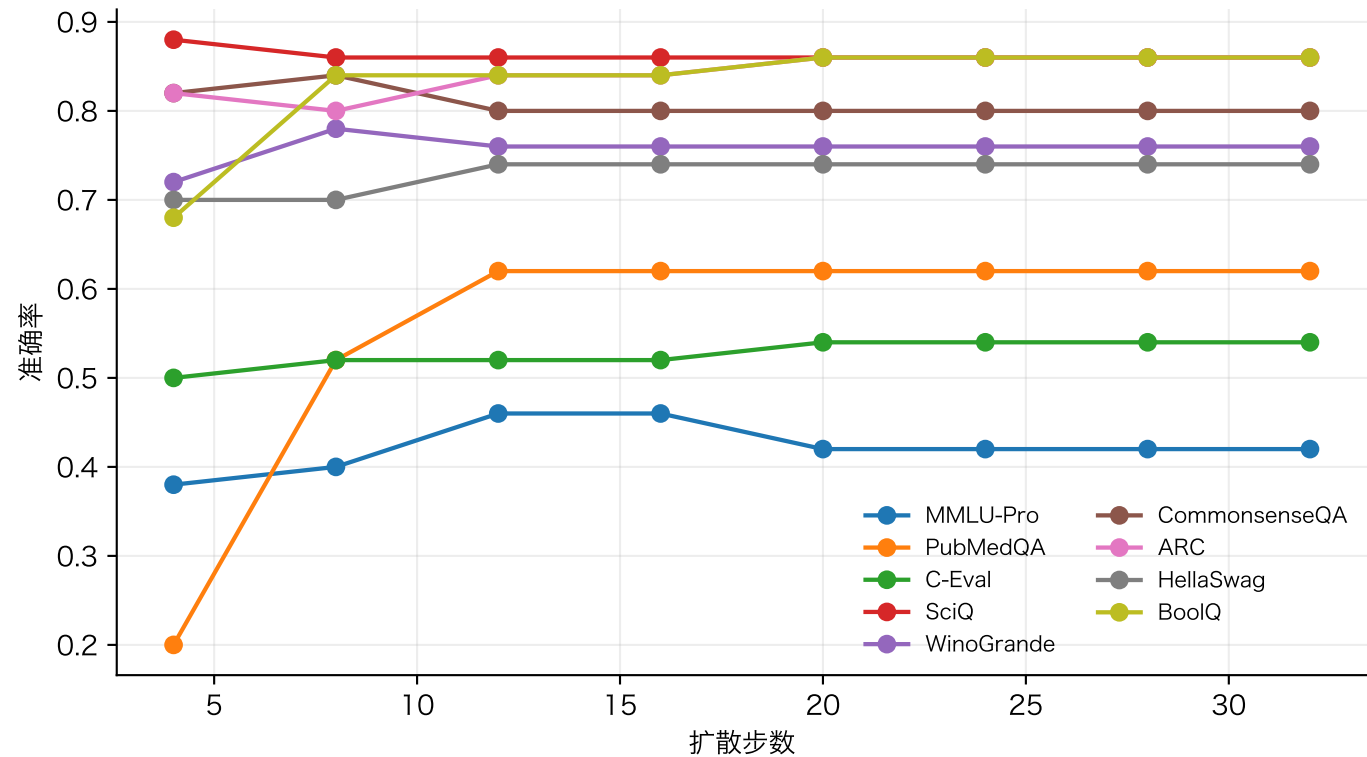
扩散步数扫描：不同任务的预算敏感性
