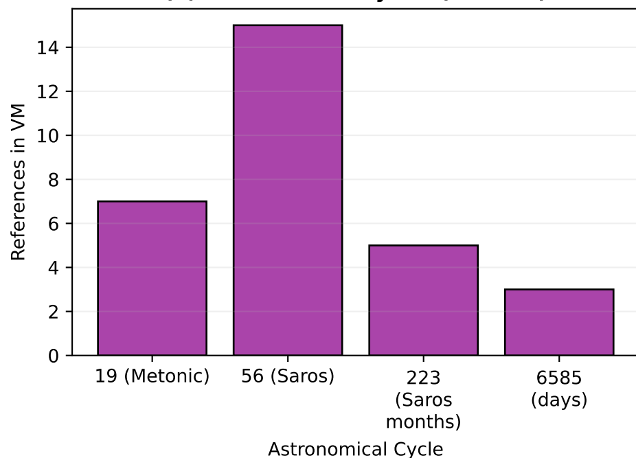
(d) Astronomical Cycles (INV-029)
