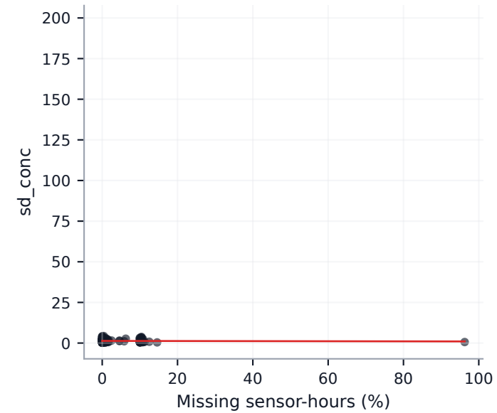
Chicago AQS
