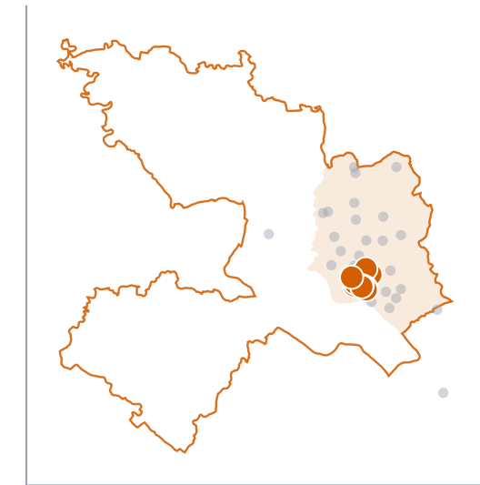
Min ESS
