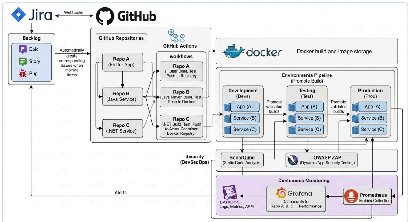
Figura 1.1: Diagrama de Tecnologías de Alto Nivel V2 — Flujo de integración, compilación y almacenamiento en registros Docker, promoción de ambientes, DevSecOps y observabilidad con bucle cerrado hacia Jira.
