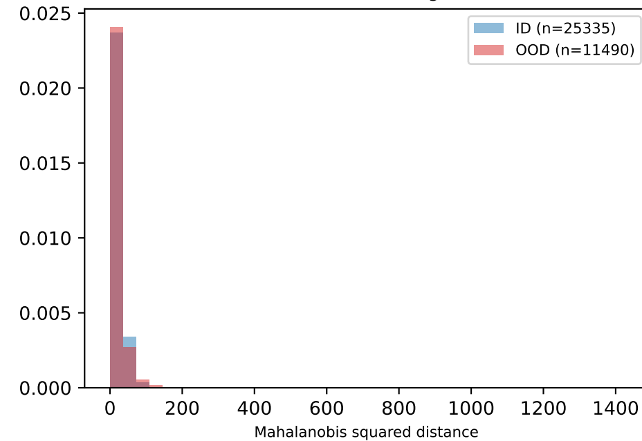
runB -- KDE
