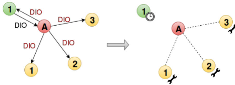
Hình 3.4 Cơ chế Version Number Attack: kẻ tấn công A giả mạo nút gốc bằng cách phát DIO với DODAGVersionNumber cao hơn, buộc toàn mạng tái cấu trúc
