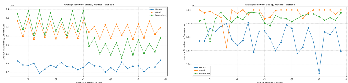
Hình 5.5 Tiêu thụ năng lượng DIS Flooding: CPU (trái) và Radio (phải)
