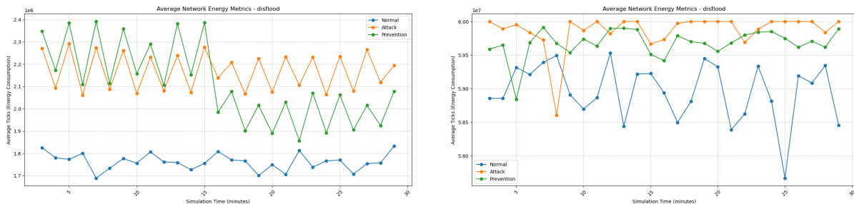
Hình 5.2 Tiêu thụ năng lượng DIS Flooding: CPU (trái) và Radio (phải)
