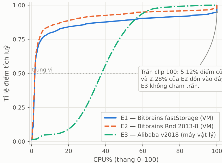
(a) ECDF, trục tuyến tính
