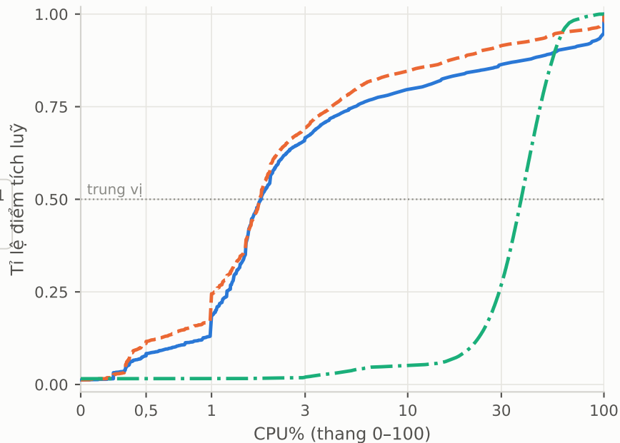
(b) ECDF, trục symlog
