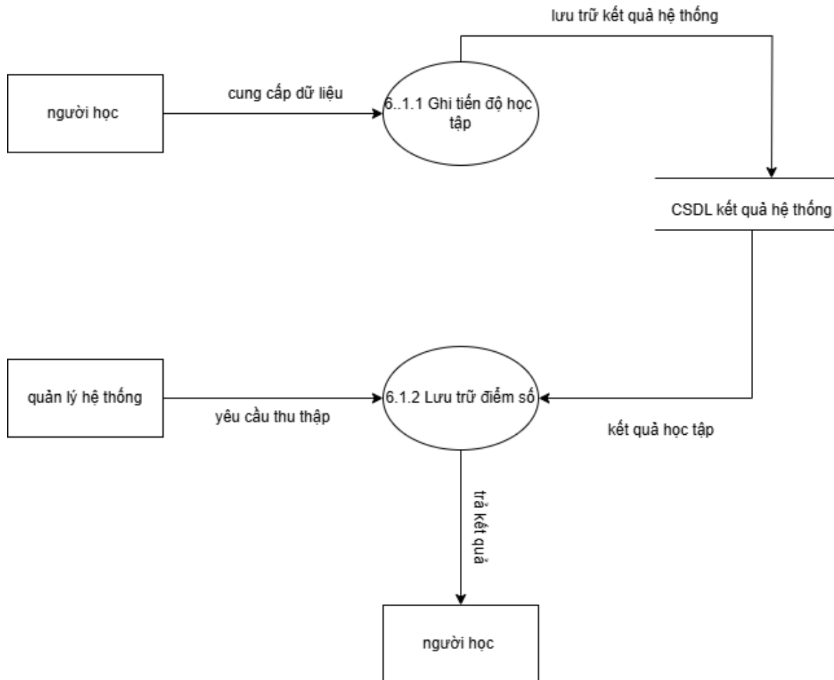
Hình 2.23 DFD cấp 2 “6.1 Thu thập dữ liệu học tập”
