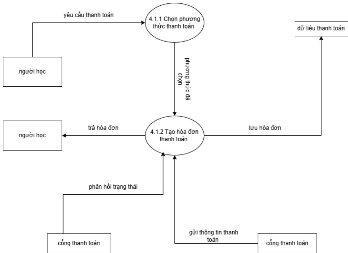
Hình 2.18 DFD cấp 2 “4.1 Yêu cầu thanh toán”
