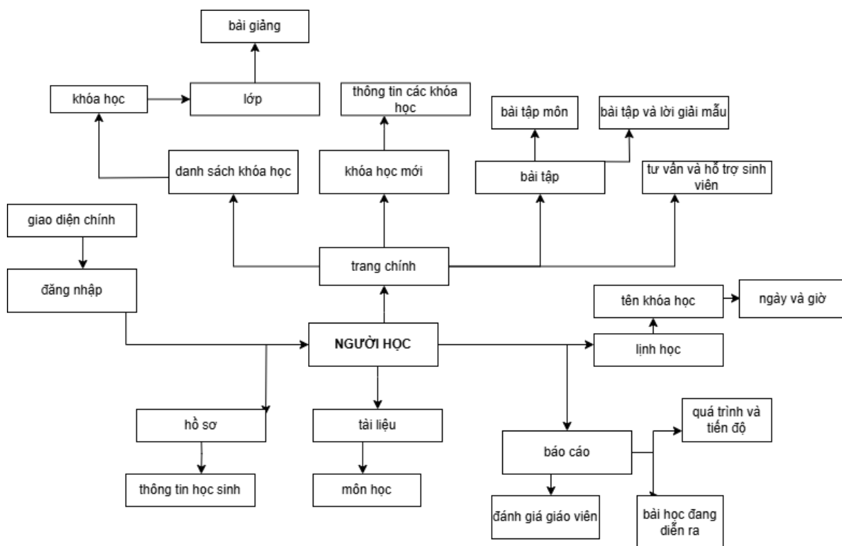
Hình 3.1 Sơ đồ hệ thống cấu trúc của Người học
