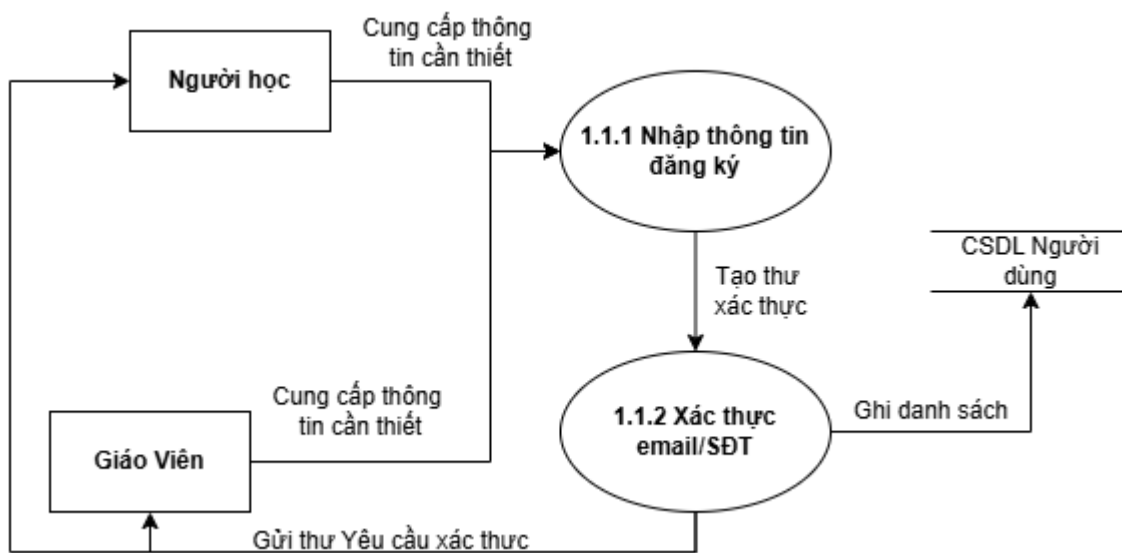
Hình 2.11 DFD cấp 2 “1.1 Đăng kí người dùng”
