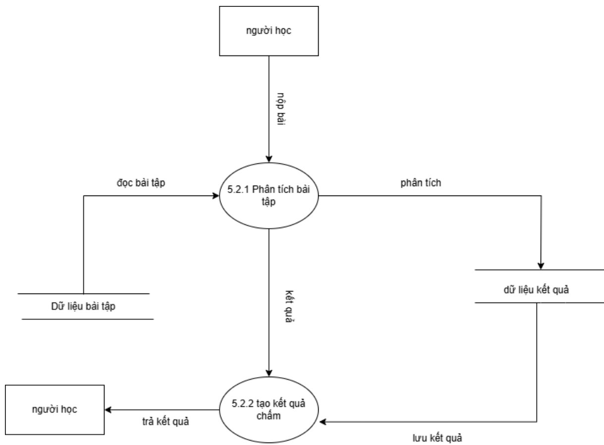
Hình 2.21 DFD cấp 2 “5.2 tự động chấm bài”
