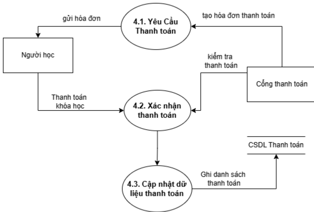
Hình 2.7 DFD mức 1 của tiến trình Quản lí thanh toán
