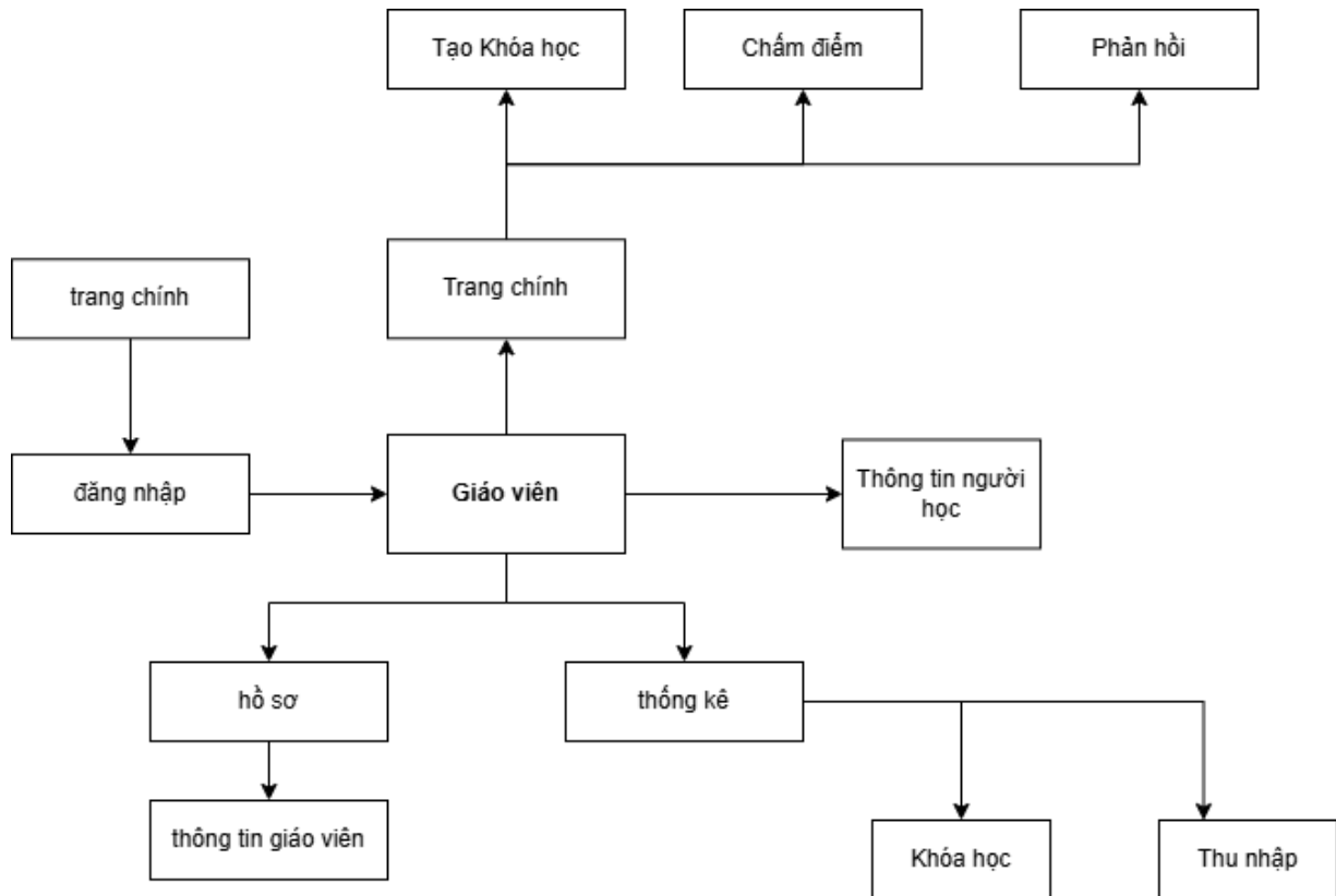
Hình 3.2 Sơ đồ hệ thống cấu trúc của Giáo viên
