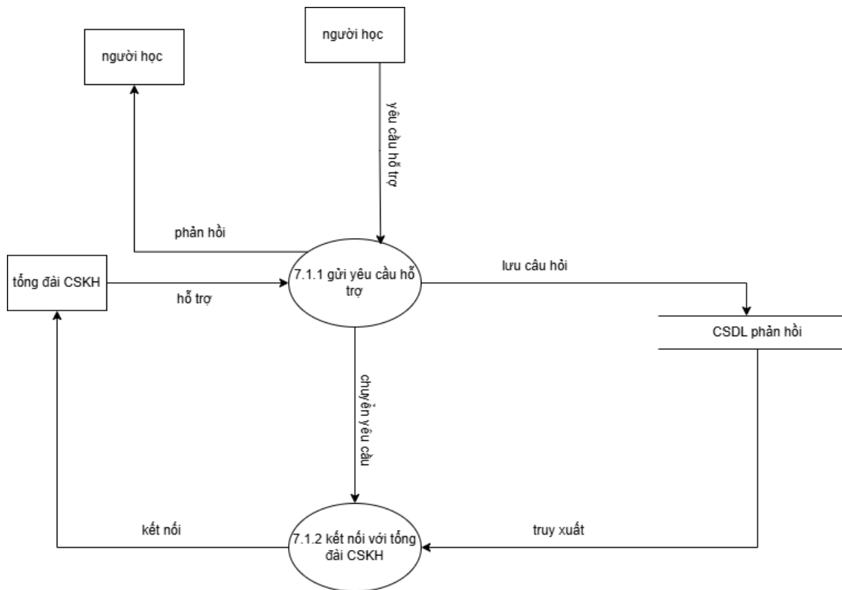
Hình 2.25 DFD cấp 2 “7.1 Hỗ trợ trực tuyến (chat/email)”
