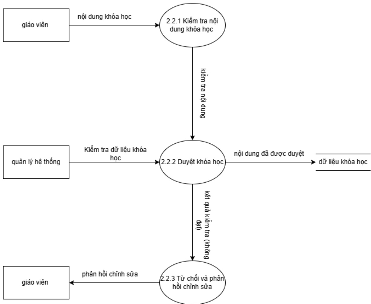
Hình 2.15 DFD cấp 2 “2.2 Kiểm duyệt khóa học”
