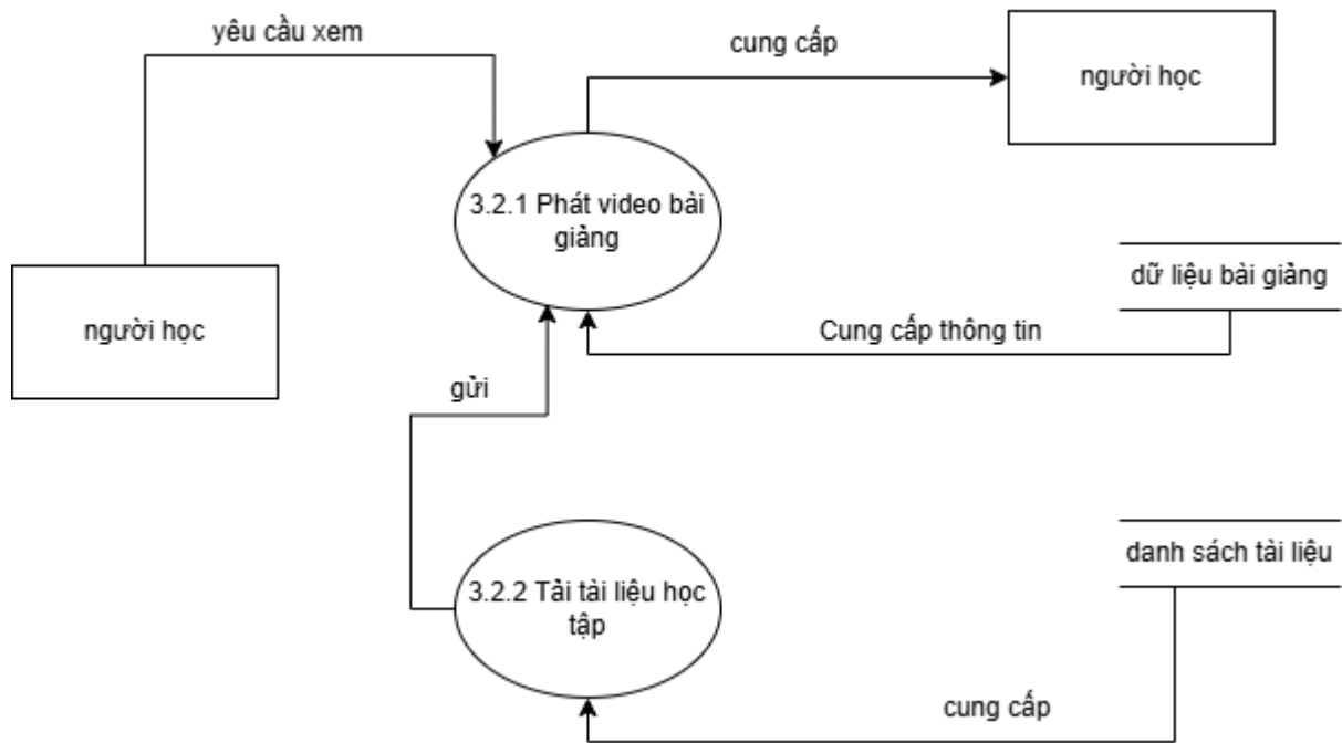
Hình 2.17 DFD cấp 2 “3.2 Xem bài giảng”
