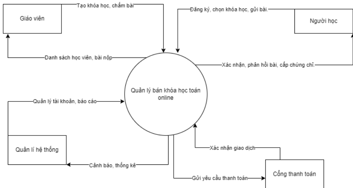
Hình 2.2 Mức ngữ cảnh của bài toán
