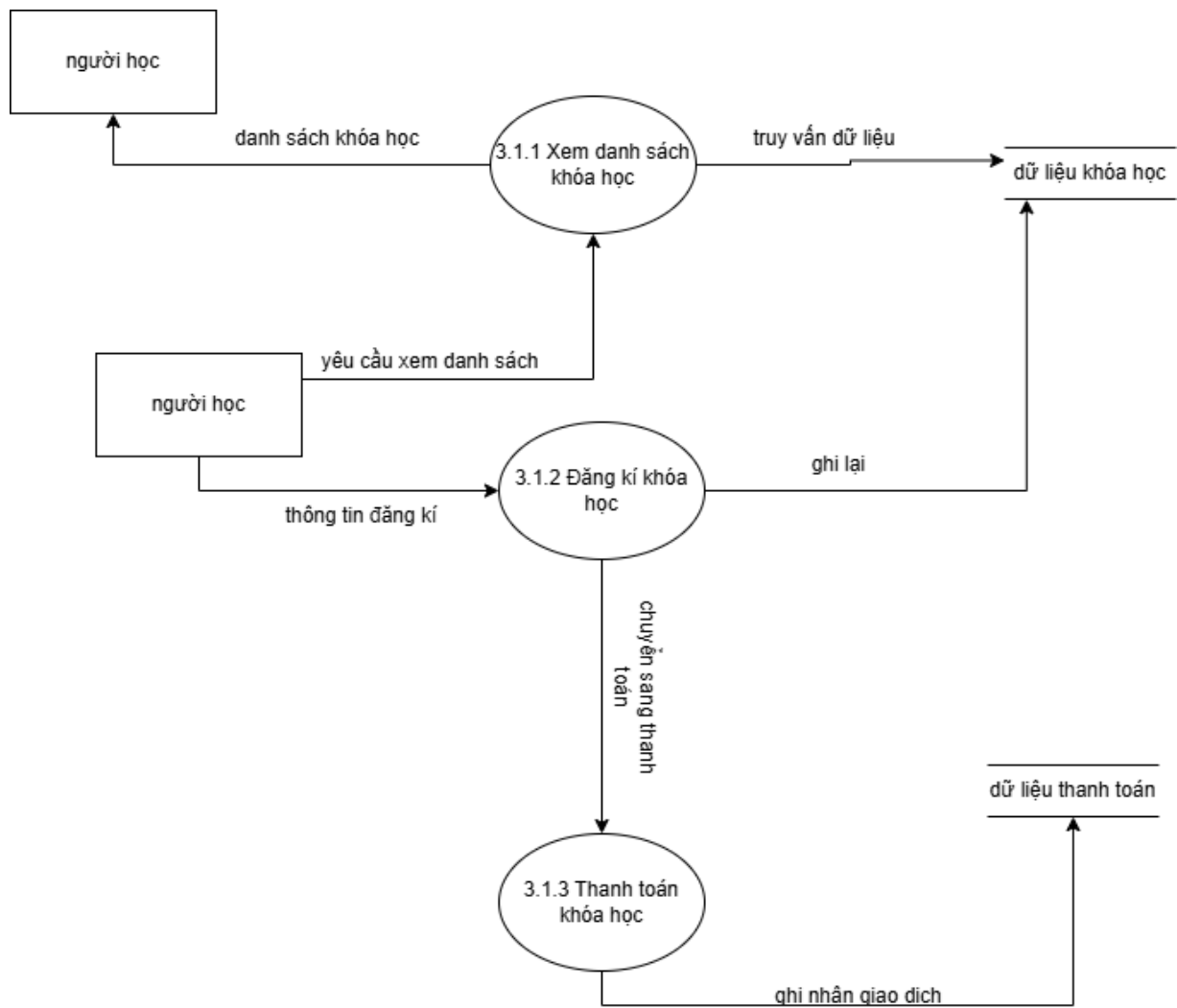
Hình 2.16 DFD cấp 2 “3.1 Chọn khóa học”
