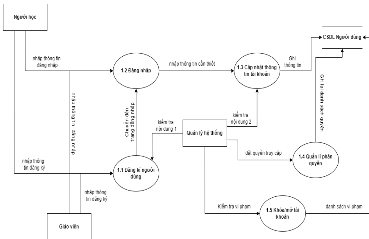
Hình 2.4 DFD mức 1 của tiến trình quản lí tài khoản
