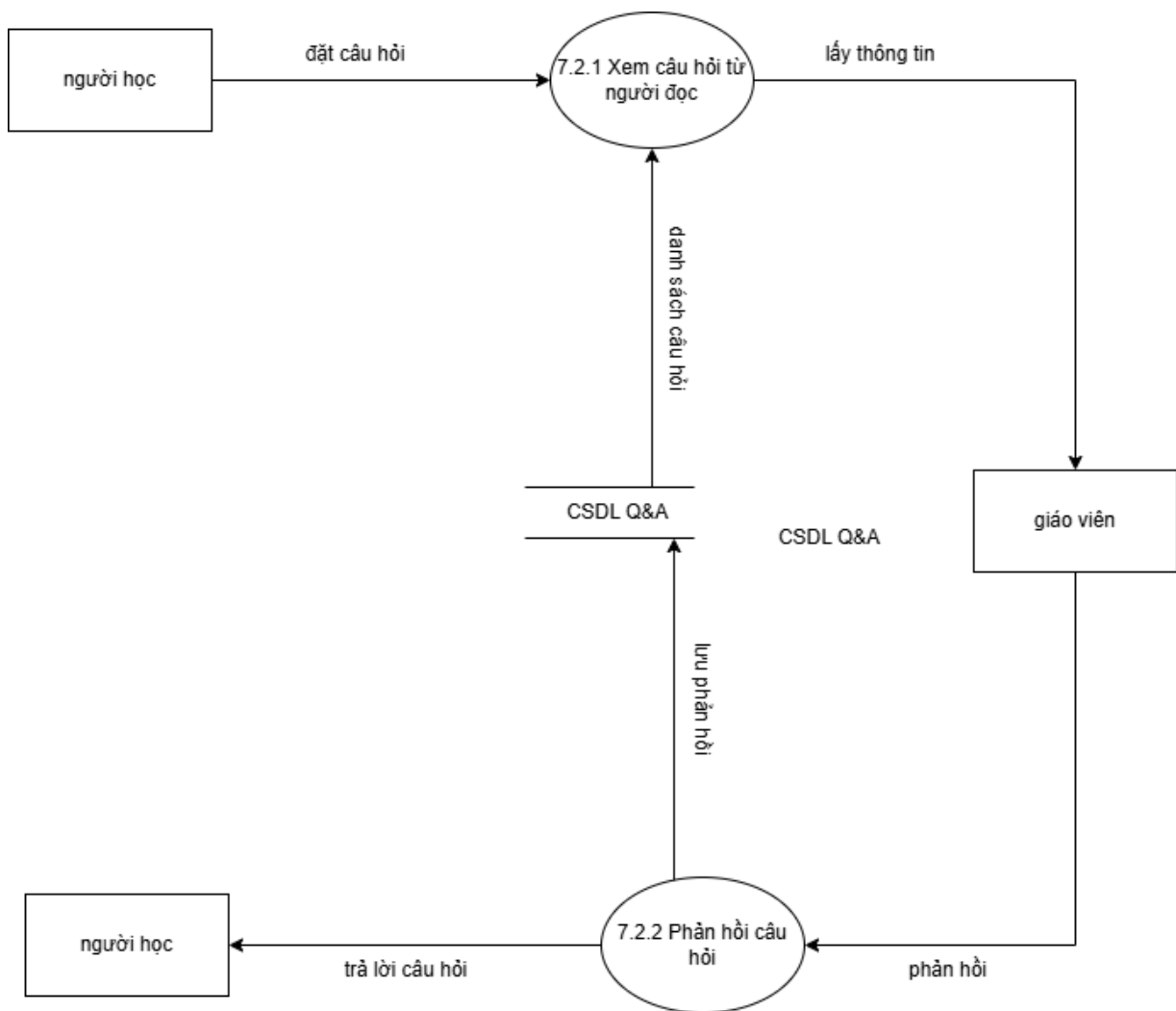
Hình 2.26 DFD cấp 2 “7.2 Trả lời câu hỏi của người học”
