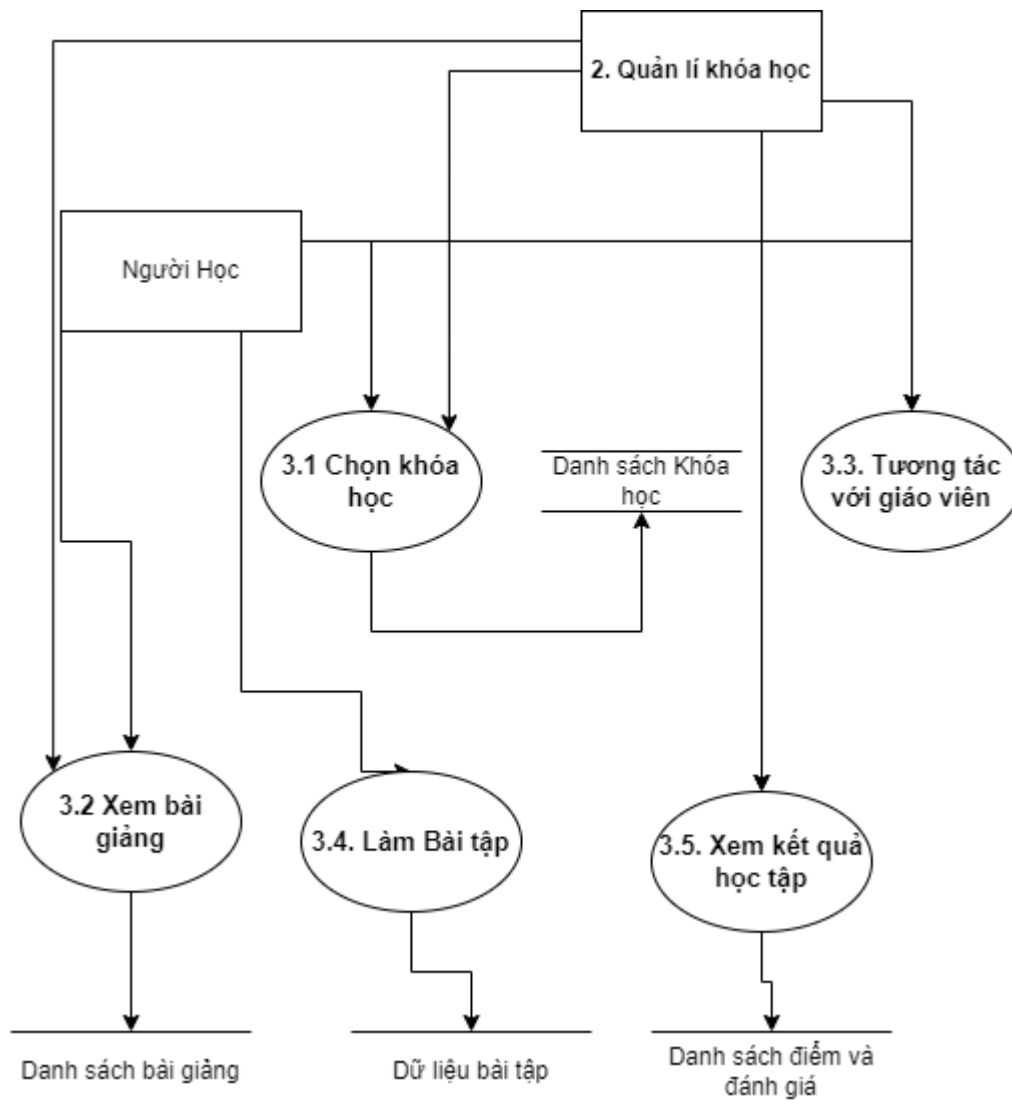
Hình 2.6 DFD mức 1 của tiến trình học tập trực tuyến
