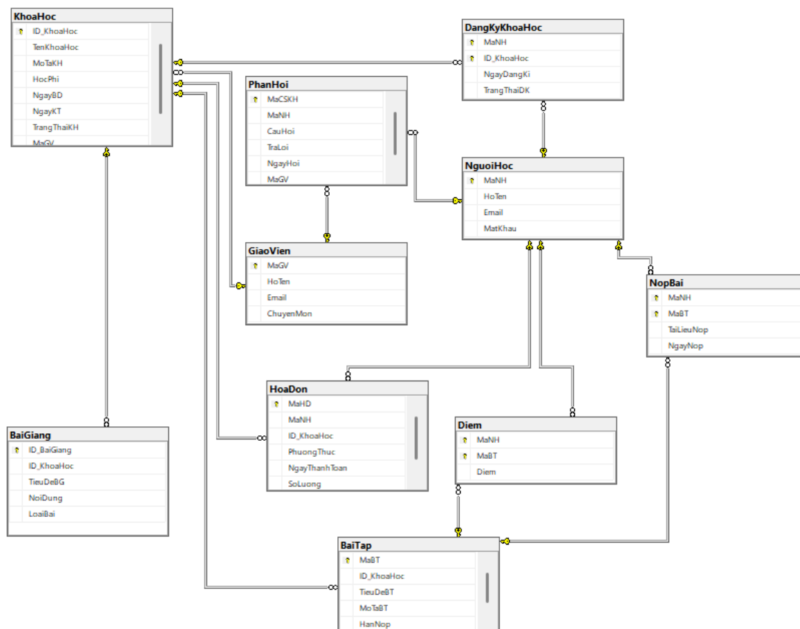
Hình 2.28 Sơ đồ RM
