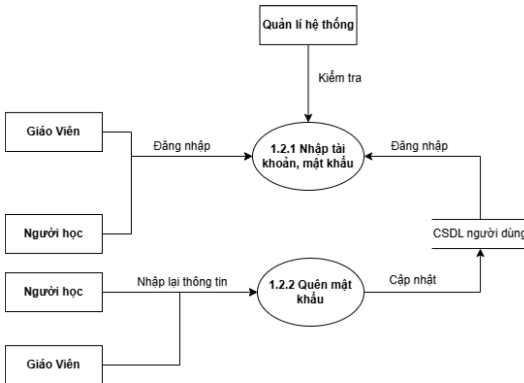
Hình 2.12 DFD cấp2 “1.2 Đăng nhập”
