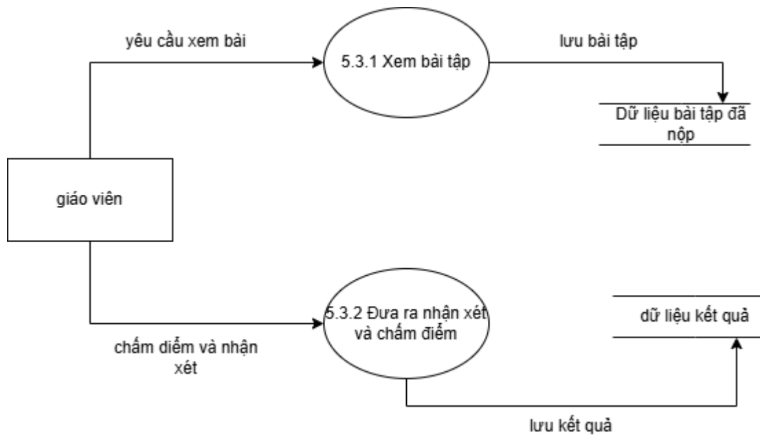
Hình 2.22 DFD cấp 2 “5.3 Giáo viên chấm bài”
