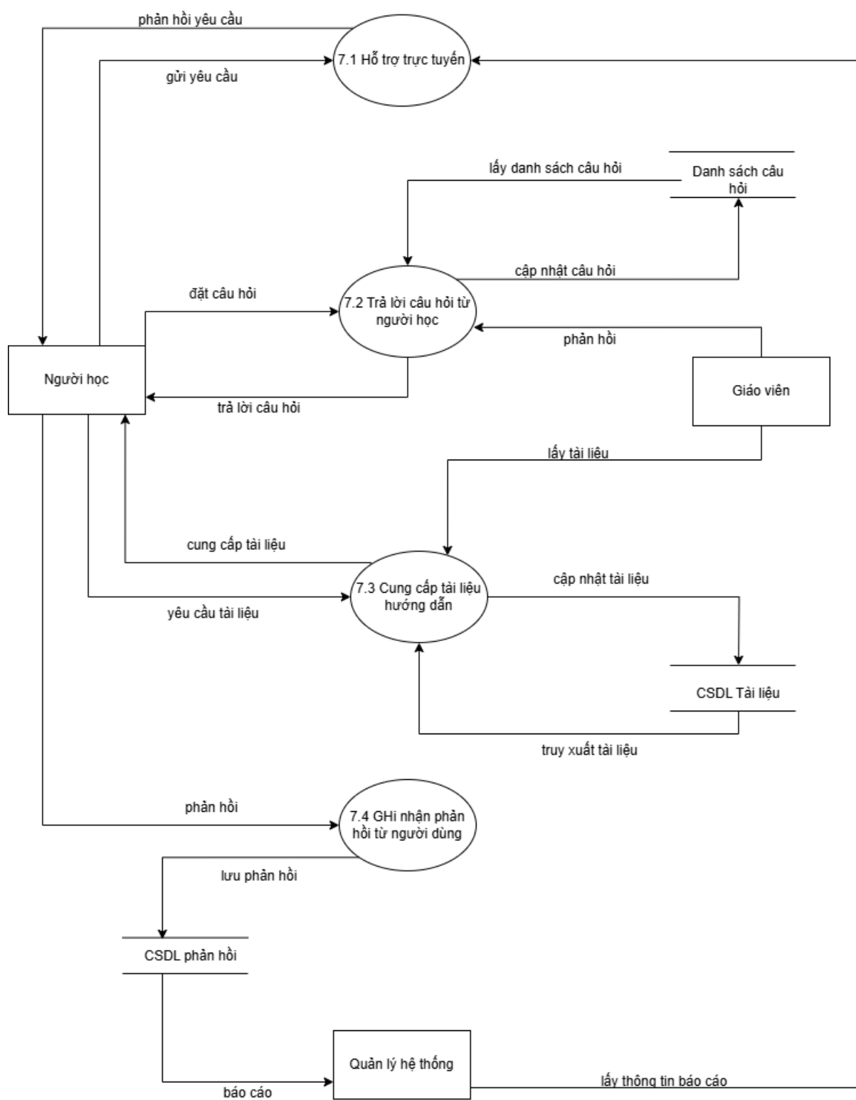
Hình 2.10 DFD mức 1 của tiến trình Hỗ trợ & Tương tác
