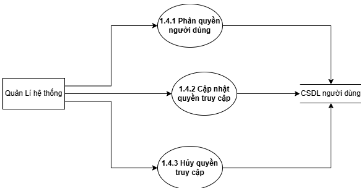
Hình 2.13 DFD Cấp 2 “1.4 Quản lí phân quyền”
