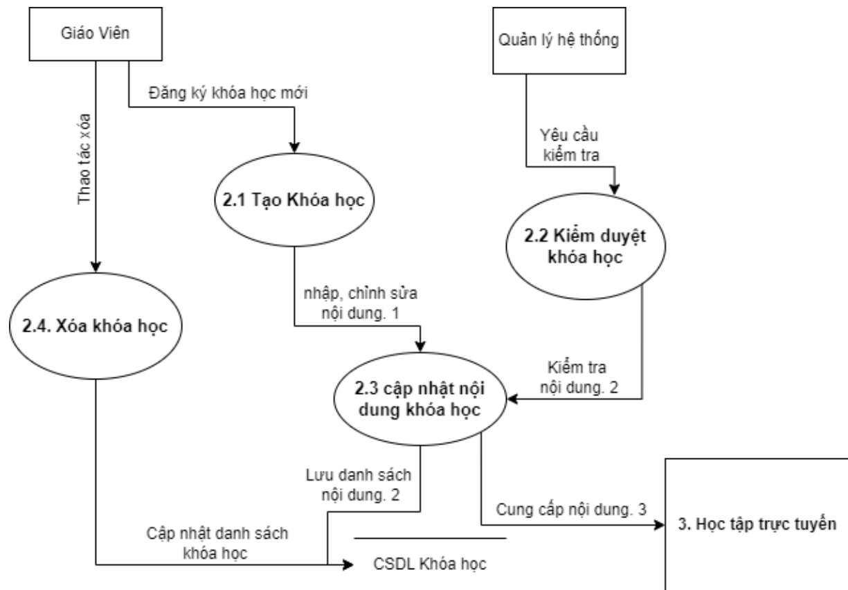
Hình 2.5 DFD mức 1 của tiến trình quản lý khóa học
