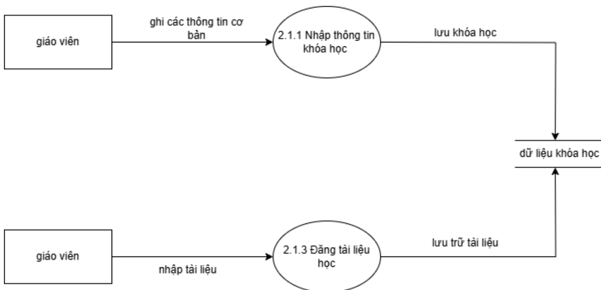
Hình 2.14 DFD cấp 2 “2.1 Tạo khóa học”
