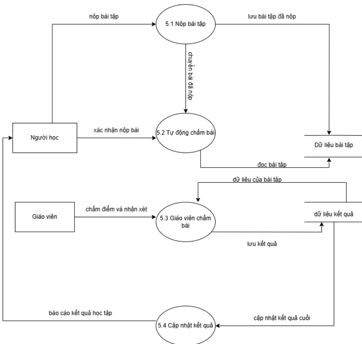
Hình 2.8 DFD mức 1 của tiến trình chấm bài và đánh giá
