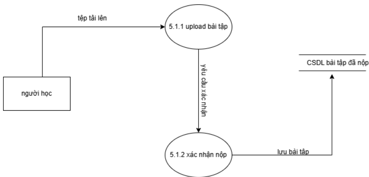
Hình 2.20 DFD cấp 2 “5.1 Nộp bài tập”
