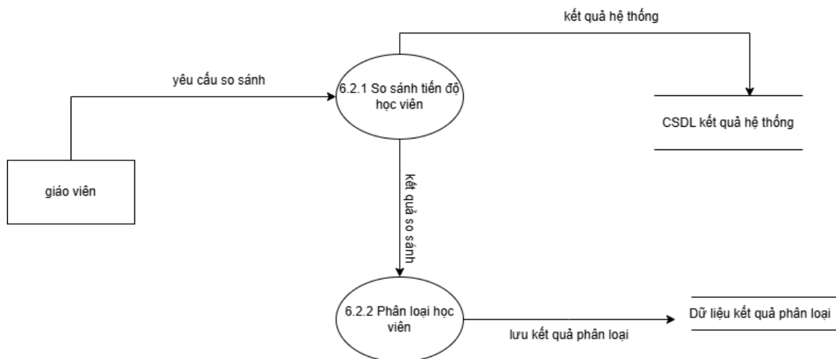
Hình 2.24 DFD cấp 2 “6.2 Phân tích tiến độ học viên”
