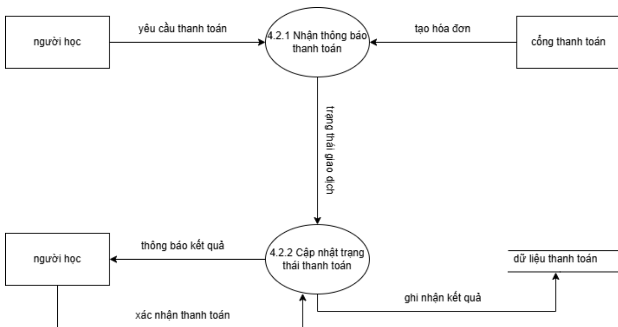
Hình 2.19 DFD cấp 2 “4.2 Xác nhận thanh toán”
