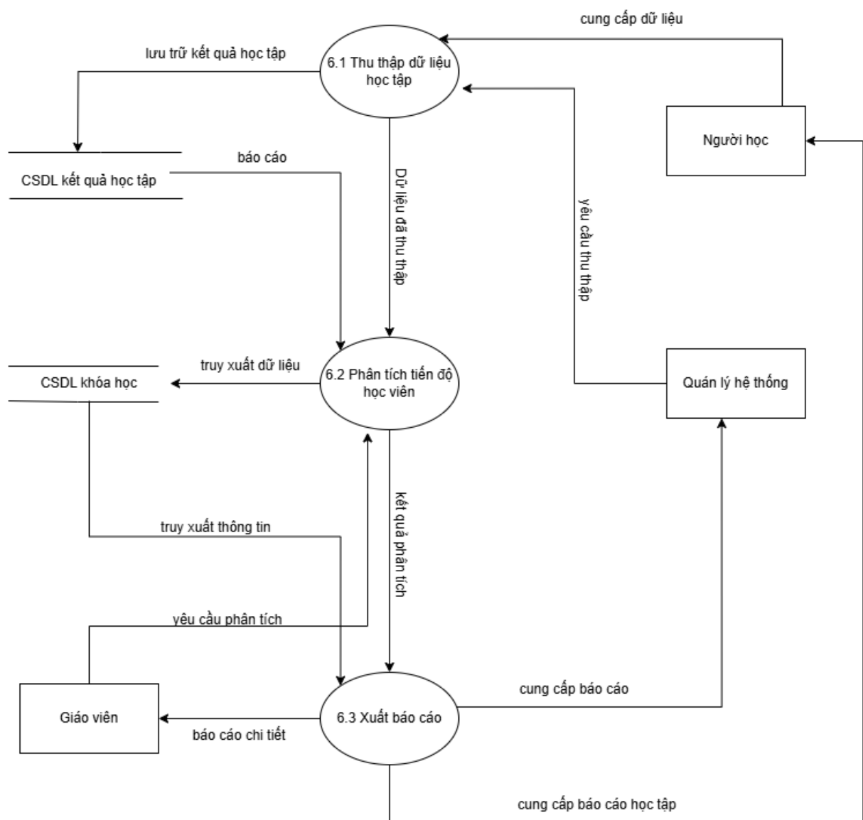
Hình 2.9 DFD mức 1 của tiến trình Báo cáo & Phân tích
