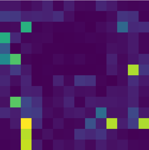
RoViT-QR W6A6
