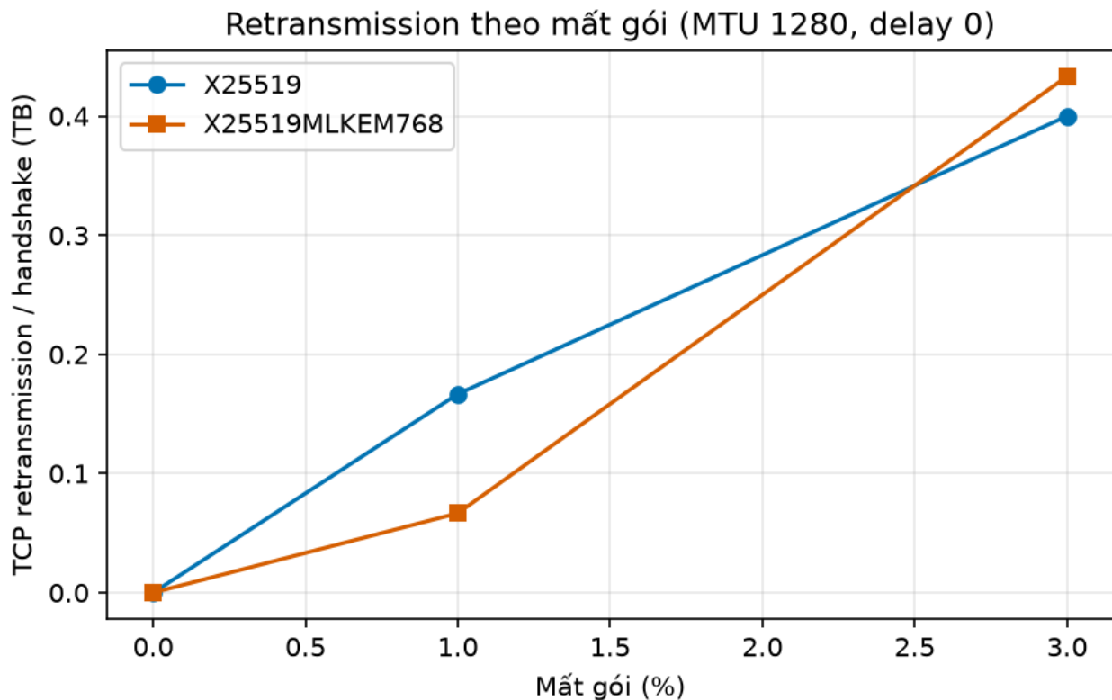
Hình 3 — Retransmission theo mất gói
