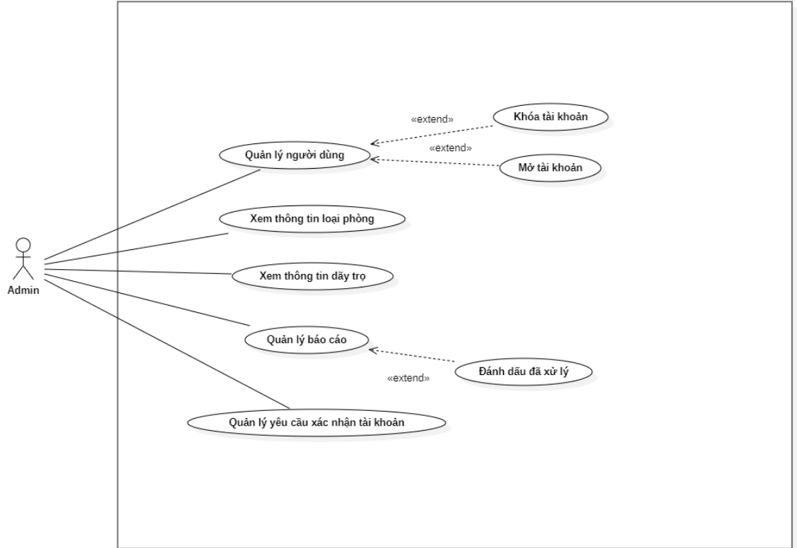
Hình 8 Sơ đồ UseCase của tác nhân “admin”
