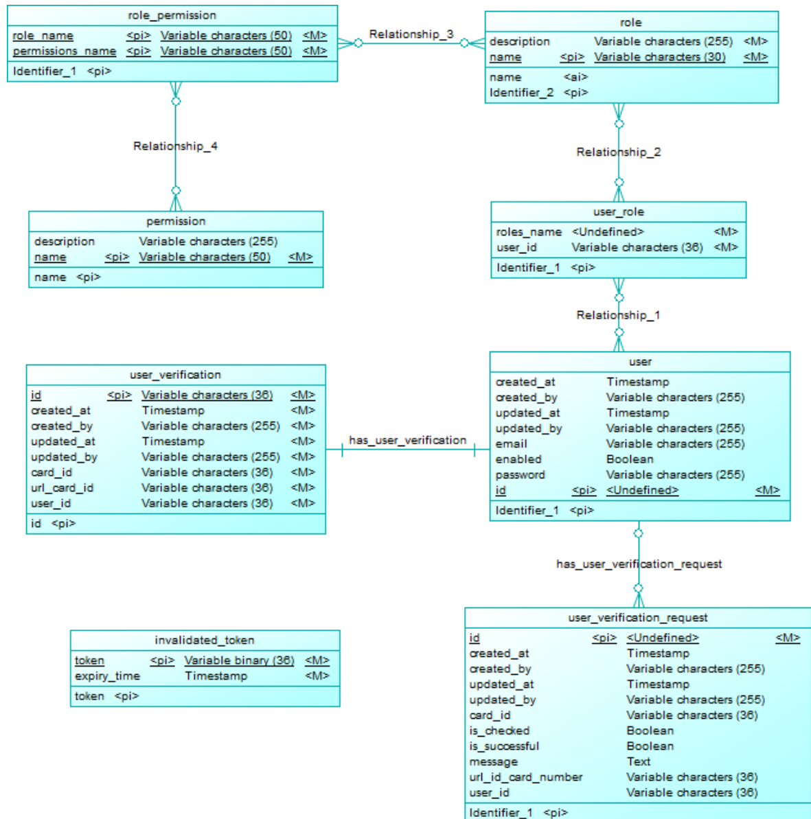
Hình 9 CDM – Mô hình mức quan niệm của Identity Service
