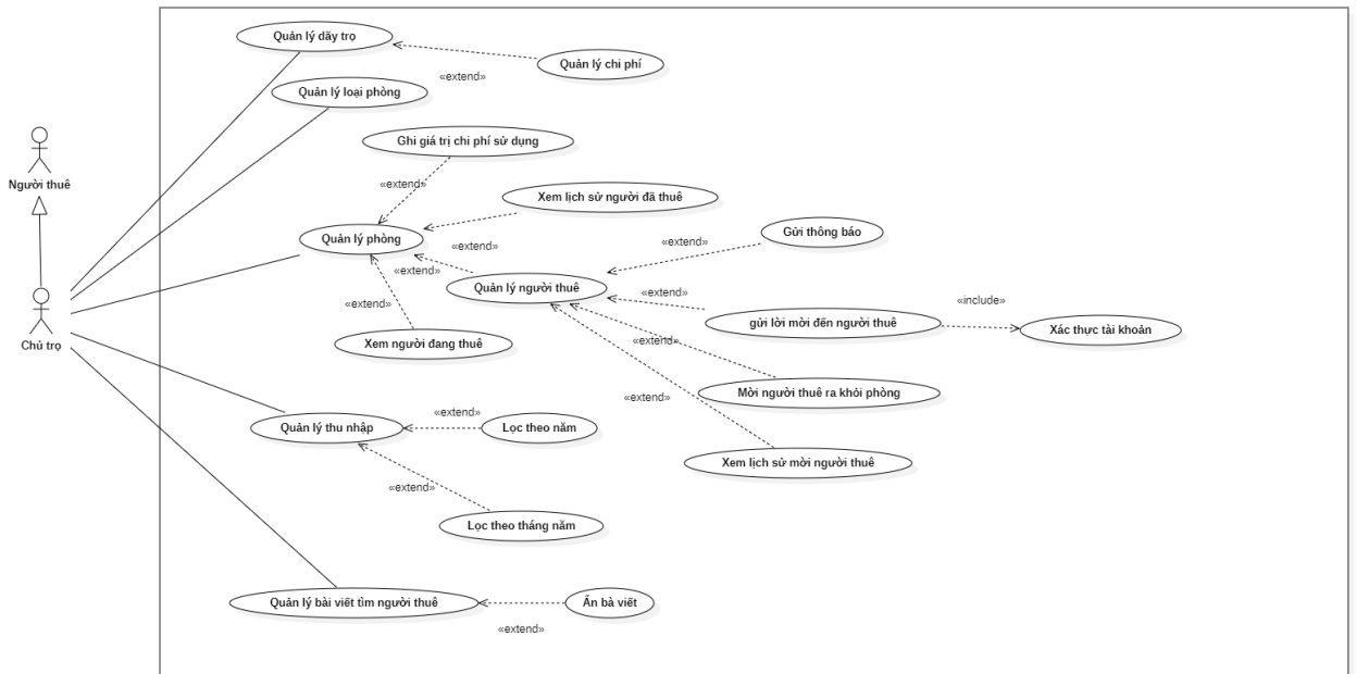
Hình 7 Sơ đồ Use Case của tác nhân “chủ trọ”
