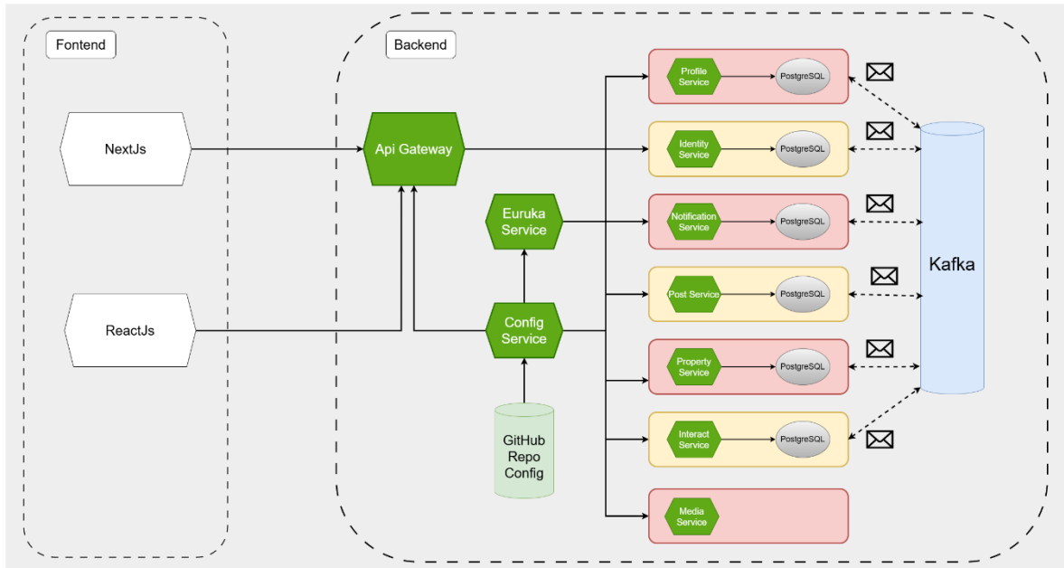
Hình 4 Kiến trúc của hệ thống
