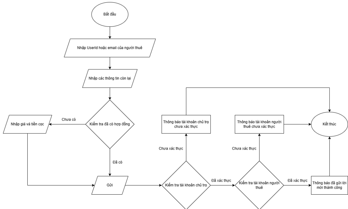
Hình 15 Chức năng mời người thuê
