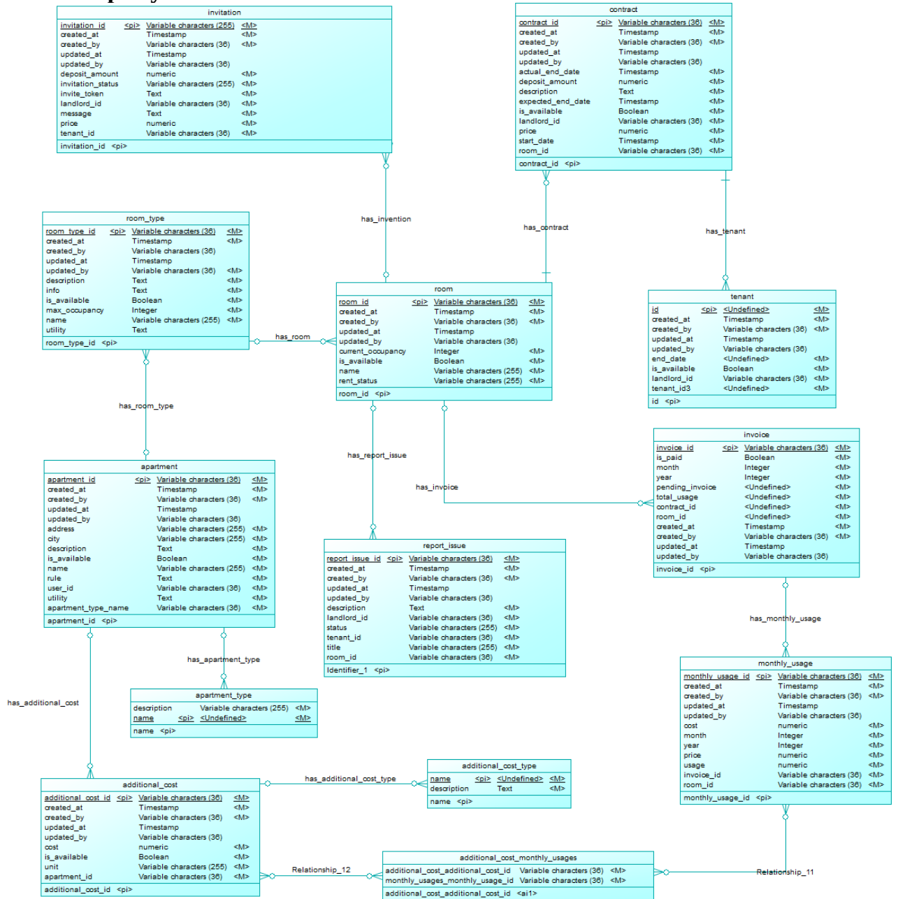
Hình 14 CDM – Mô hình mức quan niệm của Property Service
