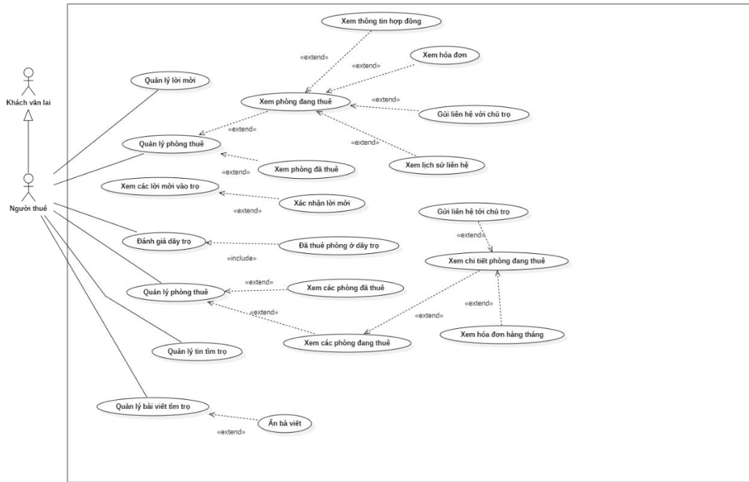
Hình 6 Sơ đồ UseCase của tác nhân “người thuê”
