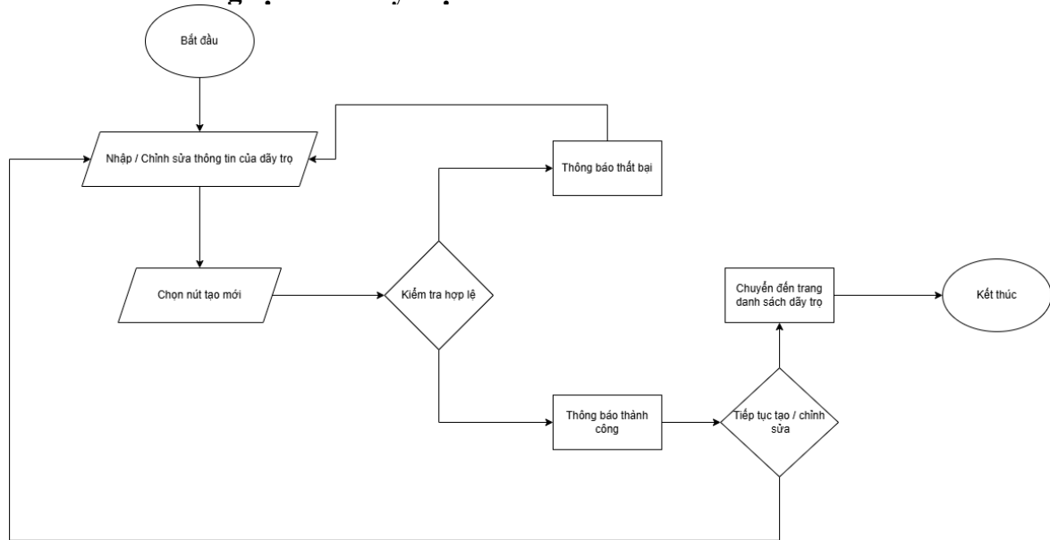
Hình 17 Chức năng tạo mới dây trọ
