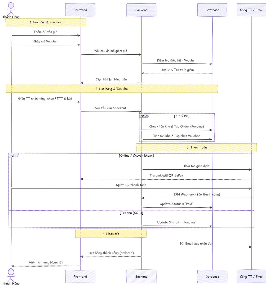
Hình 5. Quy trình giỏ hàng đặt hàng thanh toán
