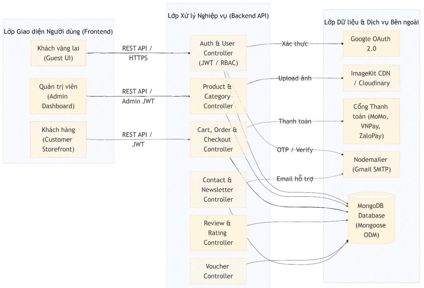
Hình 1. Kiến trúc tổng thể hệ thống TechVie
