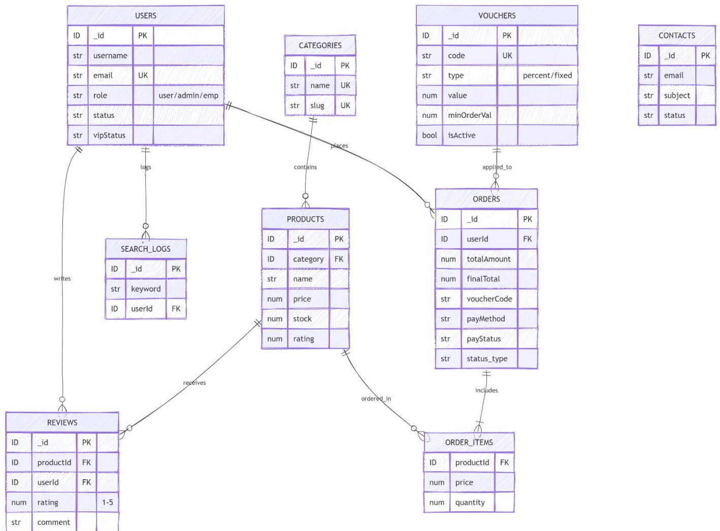
Hình 6. Sơ đồ Thực thể Liên kết (ERD) của hệ thống TechVic
