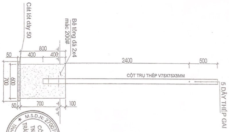
MC 2-2 - MÔNG TRỤ CỐNG M2 1/25
