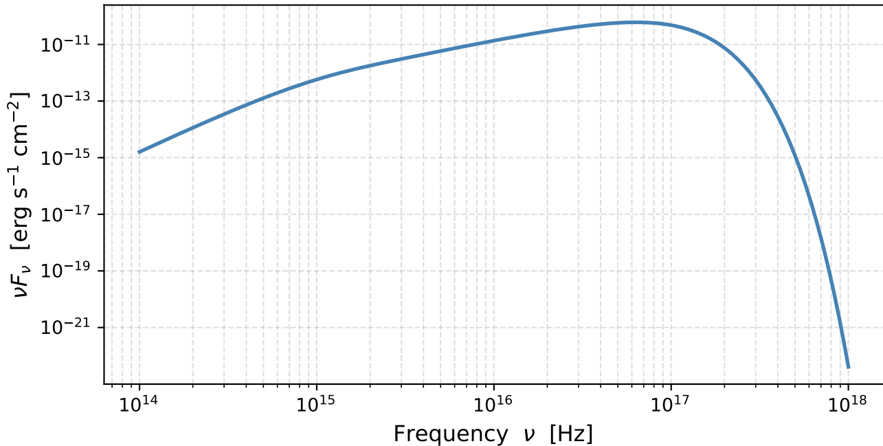
Multi-colour blackbody SED — 10 M_{\odot} BH, \dot{M} = 10^{16} \text{ g s}^{-1} , D_L = 10 \text{ kpc}
