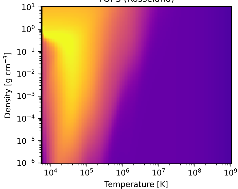
TOPS (Rosseland)
