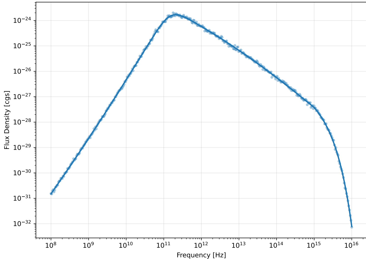
Synchrotron SED (Cooling + SSA)
