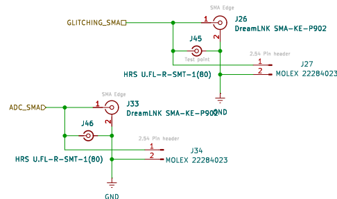
SMA EDGE CONNECTOR
