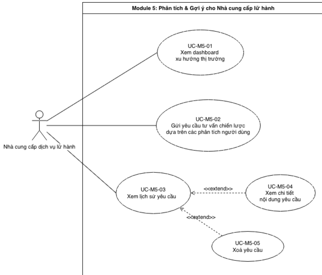
Hình 8: Use case diagram Phân tích & gợi ý cho nhà cung cấp
