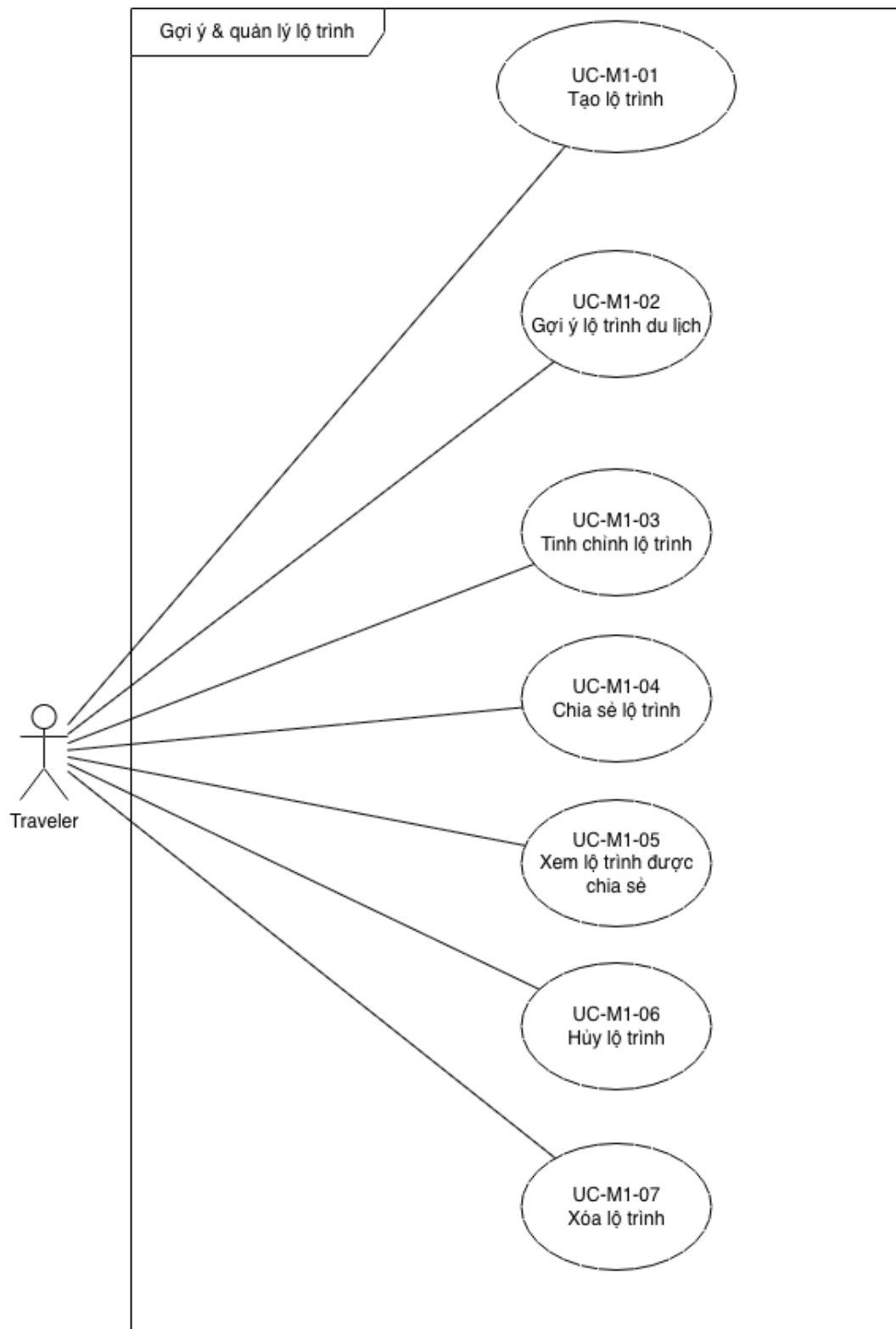
Hình 4: Use case diagram Gợi ý & quản lý lộ trình
