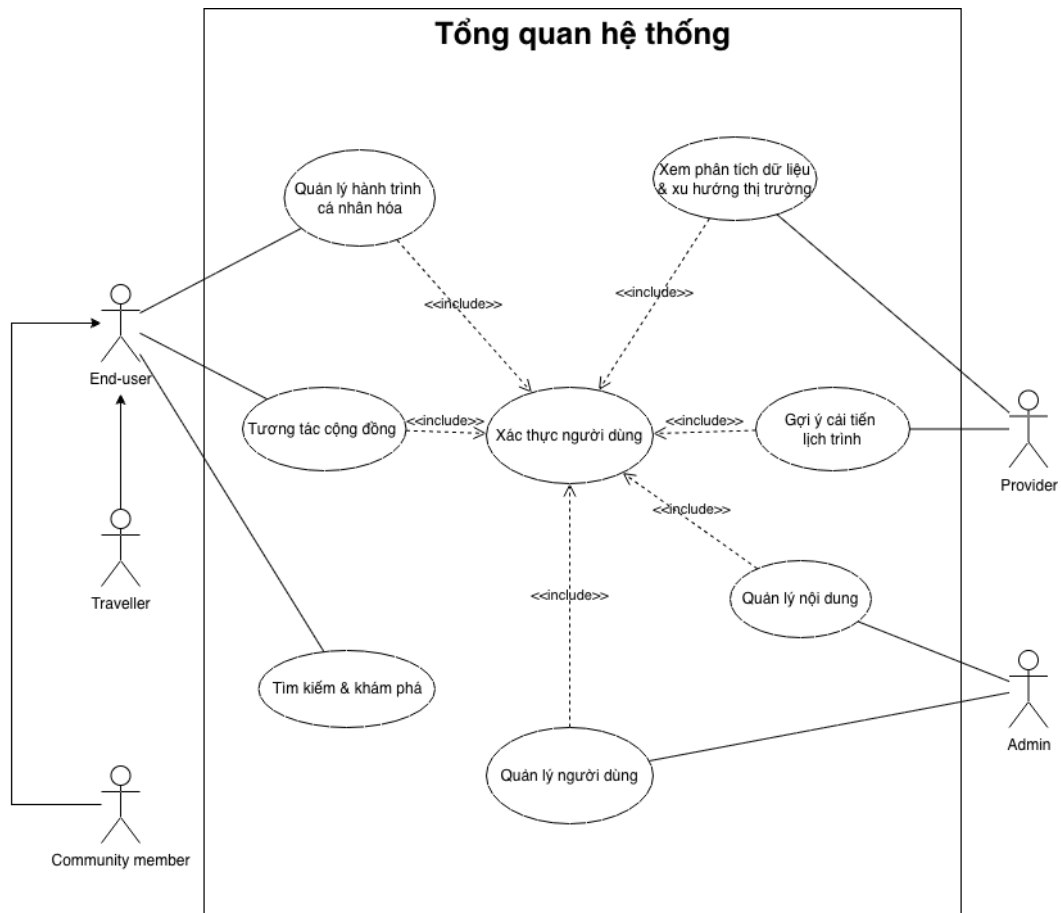
Hình 3: Use case diagram cho tổng quan hệ thống
