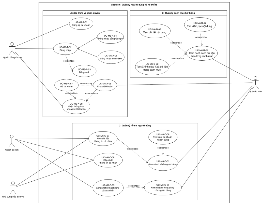
Hình 9: Use case diagram Quản trị hệ thống & người dùng
