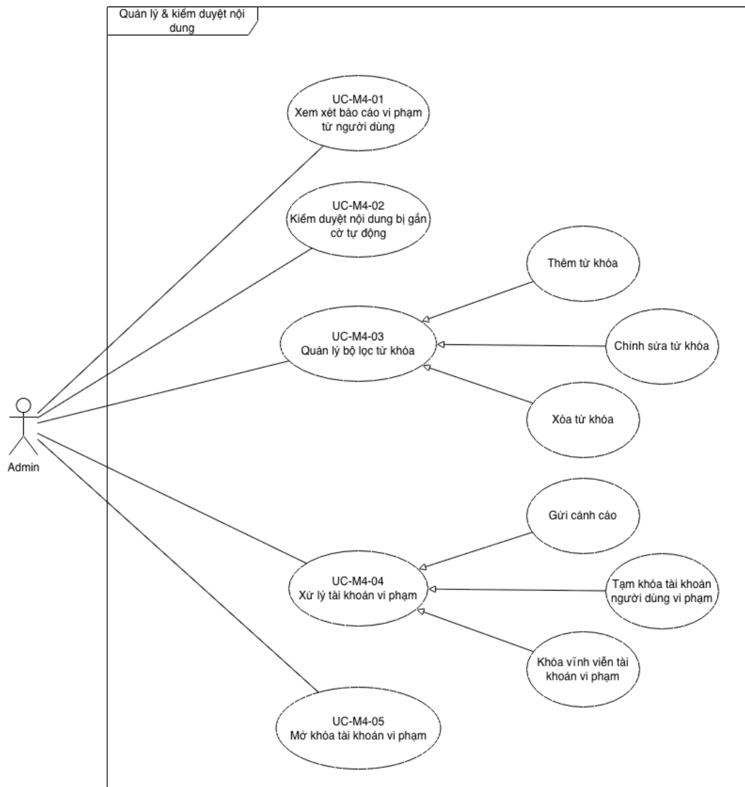
Hình 7: Use case diagram Quản lý & kiểm duyệt nội dung
