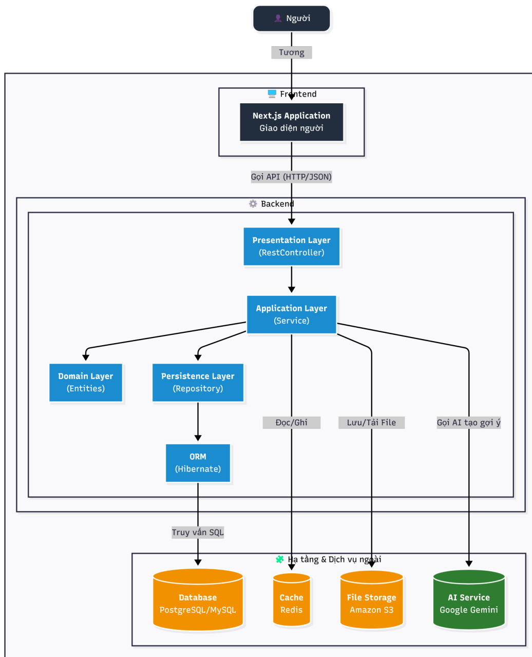
Hình 10: Kiến trúc hệ thống
