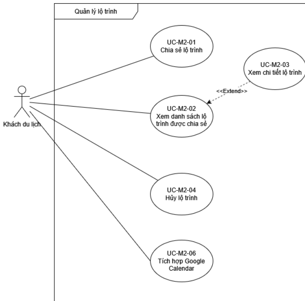
Hình 9: Use case diagram cho Module 2: Quản lý lộ trình
