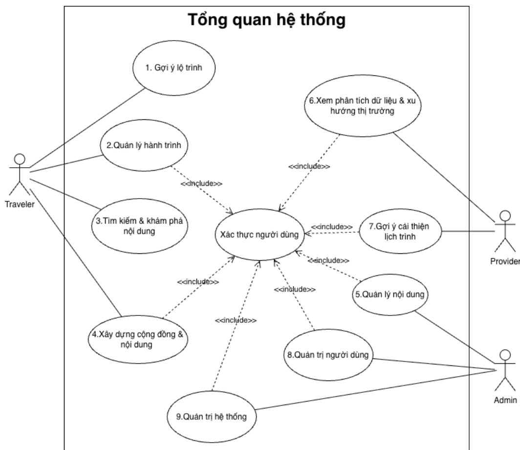
Hình 7: Use case diagram cho tổng quan hệ thống
