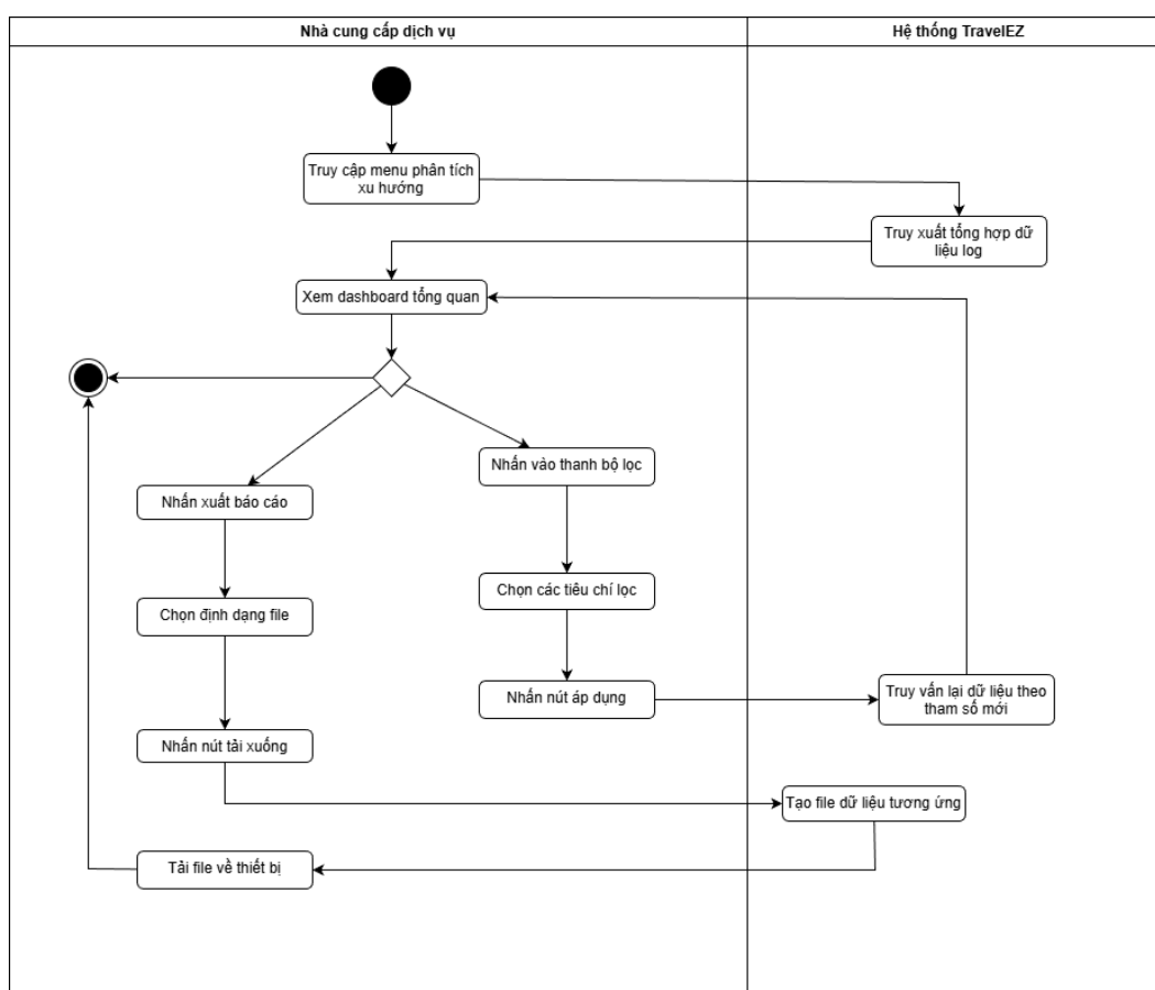
Hình 5: Activity diagram: Quy trình phân tích xu hướng thị trường
