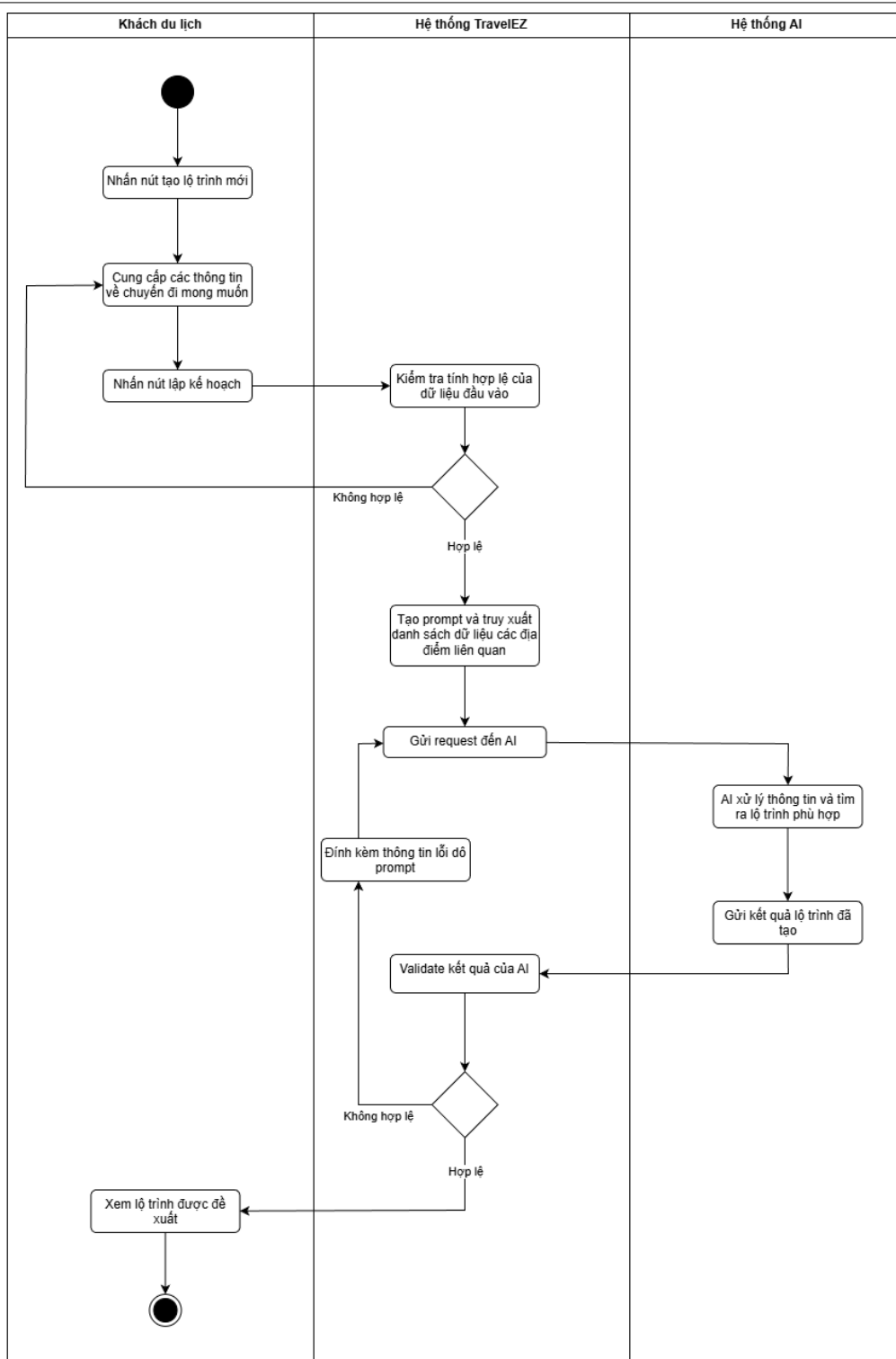
Hình 3: Activity diagram: Quy trình gợi ý lộ trình cá nhân hóa
