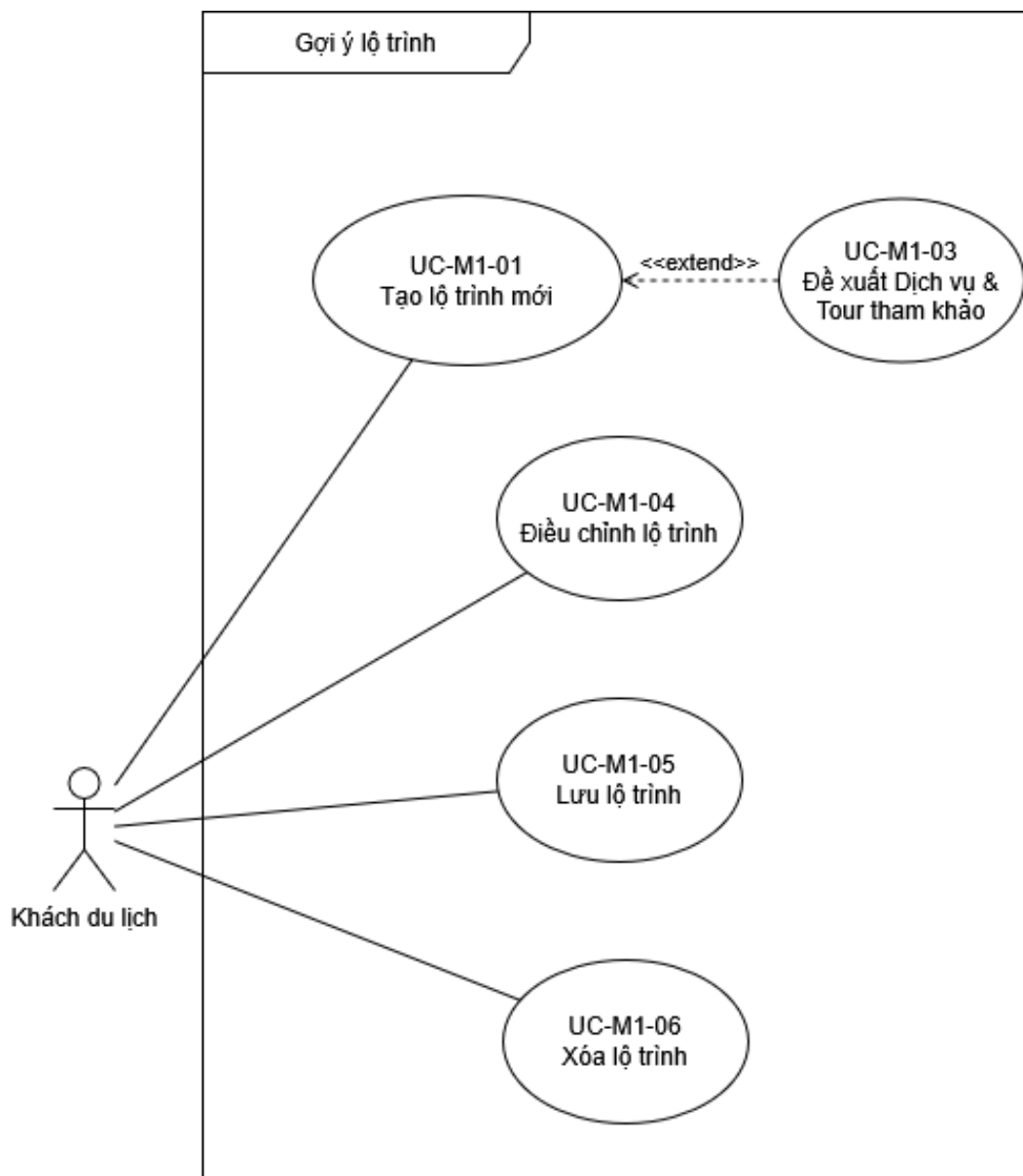
Hình 8: Use case diagram cho Module 1: Gợi ý lộ trình
