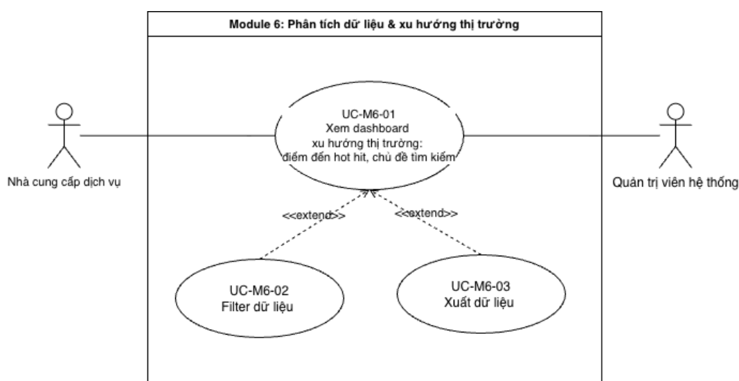
Hình 13: Use case diagram cho Module 6: Phân tích dữ liệu & xu hướng thị trường
