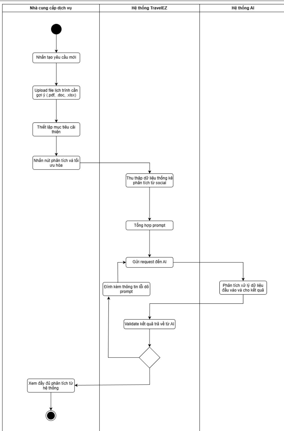
Hình 6: Activity diagram: Quy trình phân tích lịch trình cải thiện
