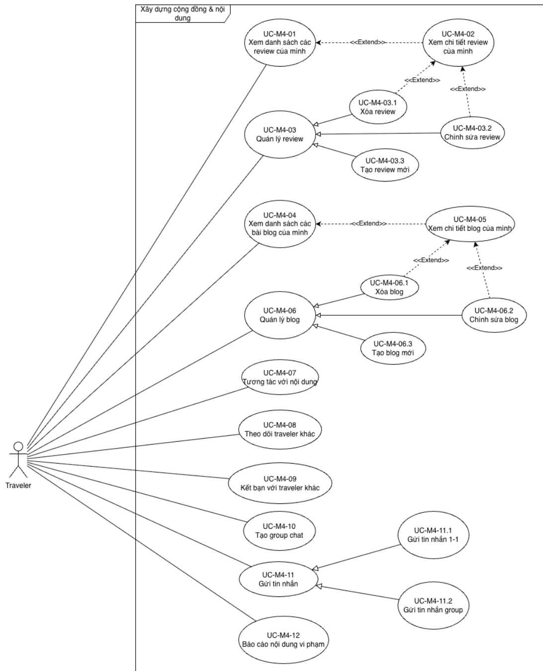
Hình 8: Use case diagram Xây dựng cộng đồng
