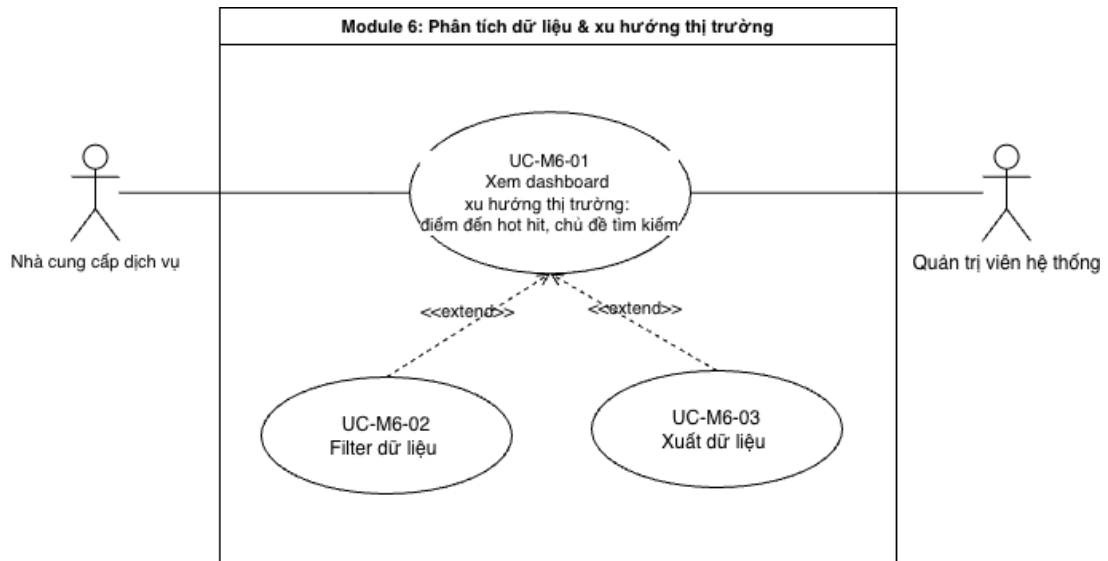
Hình 10: Use case diagram Phân tích dữ liệu và xu hướng cho nhà cung cấp dịch vụ
