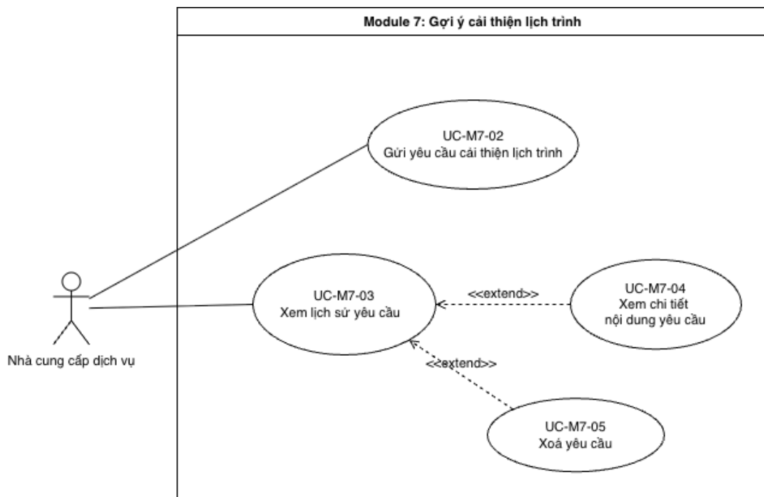
Hình 11: Use case diagram Gợi ý cải thiện lịch trình
