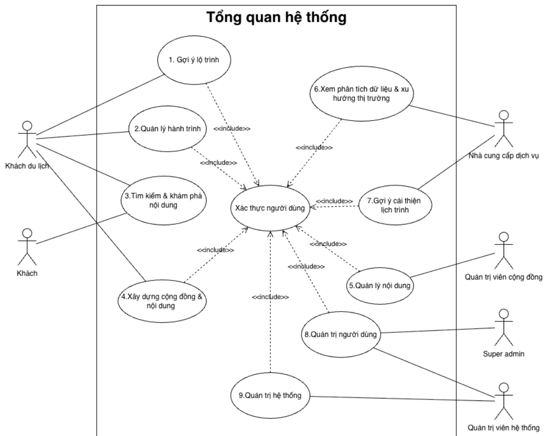
Hình 4: Use case diagram cho tổng quan hệ thống
