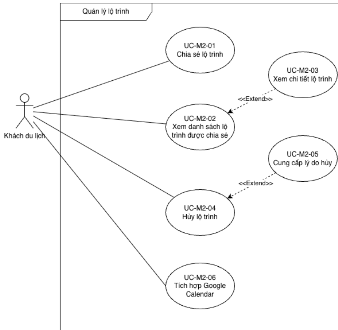
Hình 6: Use case diagram Quản lý lộ trình
