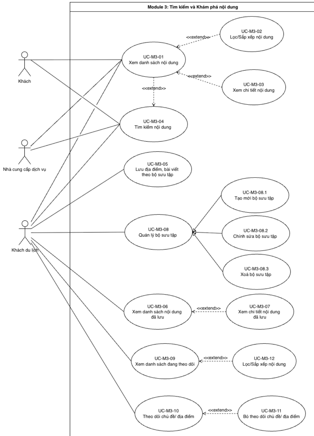
Hình 7: Use case diagram Tìm kiếm và khám phá
