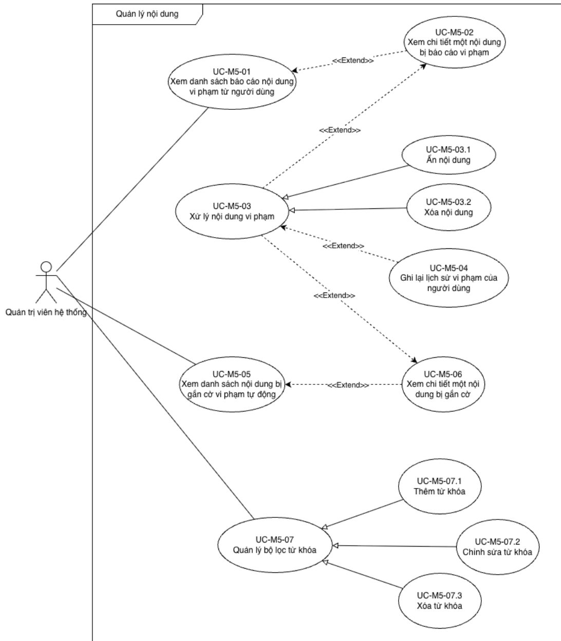
Hình 9: Use case diagram Quản lý nội dung
