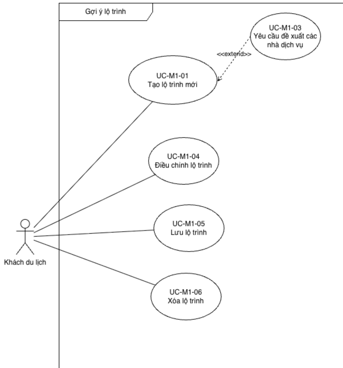
Hình 5: Use case diagram Gợi ý lộ trình
