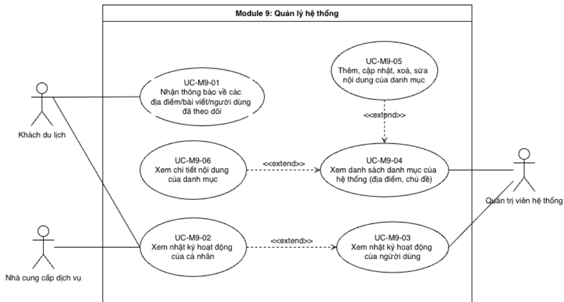
Hình 13: Use case diagram Quản trị hệ thống
