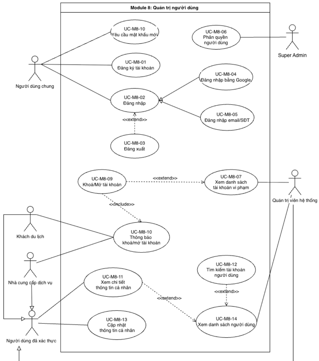
Hình 12: Use case diagram Quản trị người dùng
