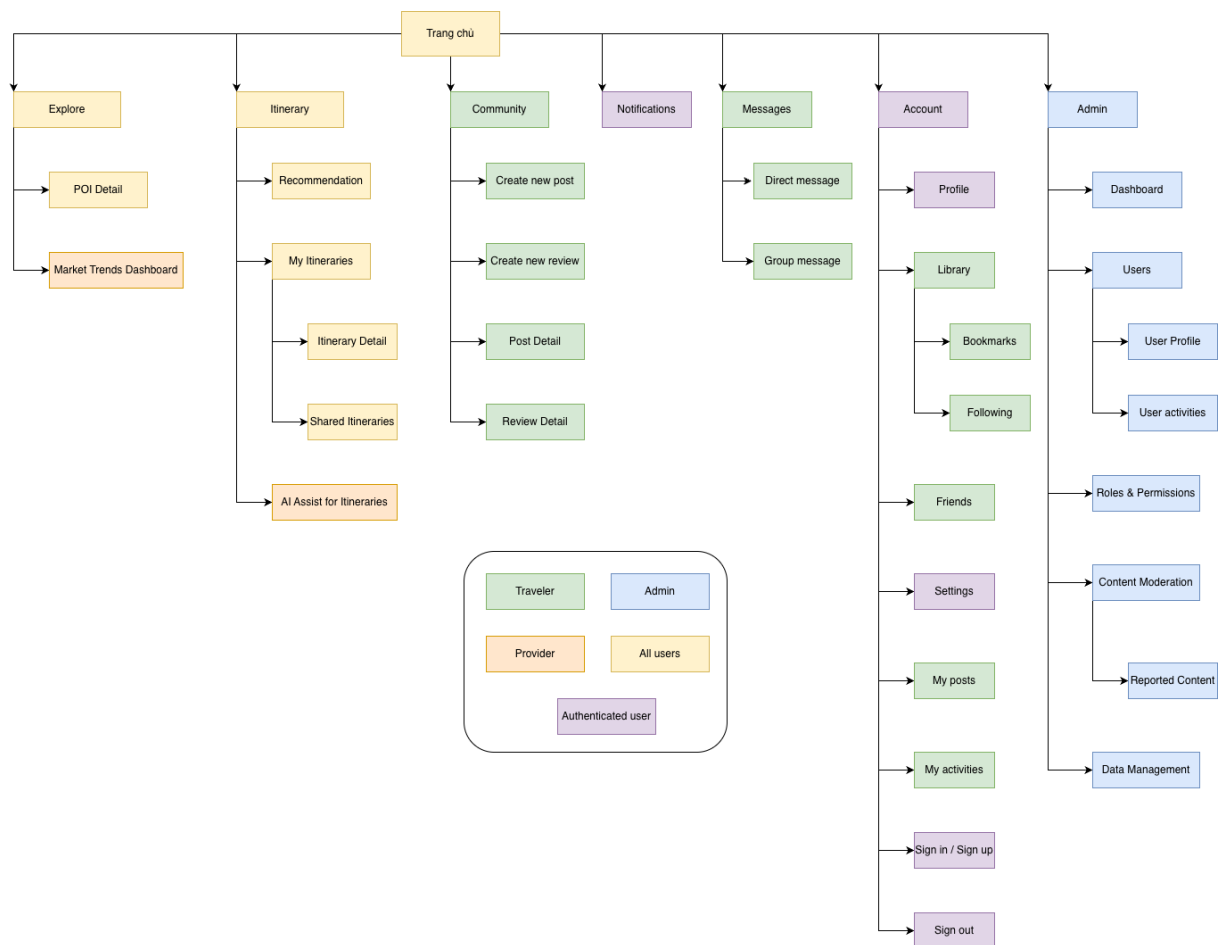
Hình 15: Sitemap của hệ thống TravelEZ
