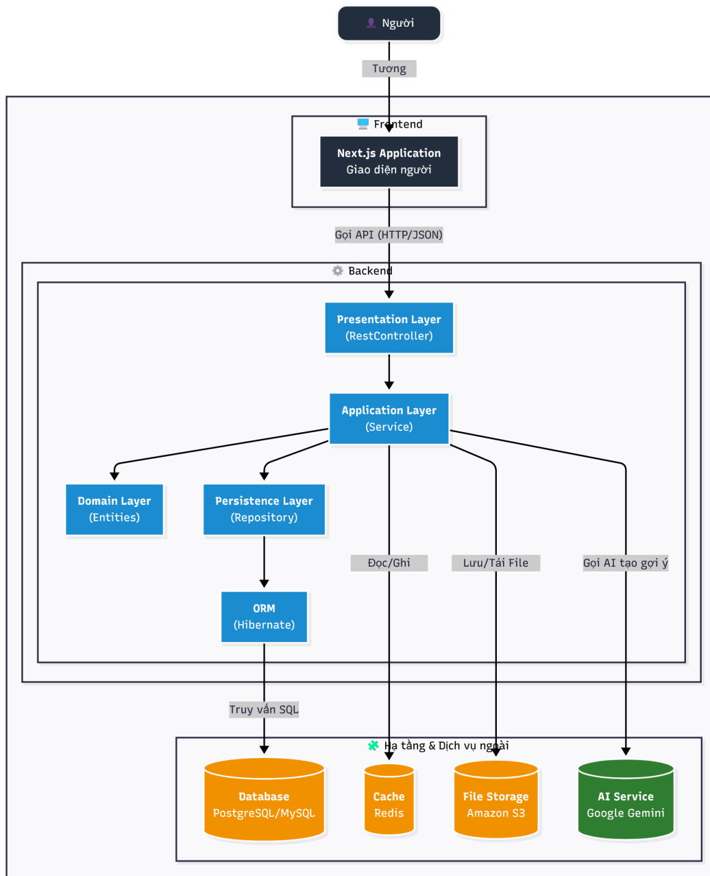
Hình 12: Kiến trúc hệ thống
