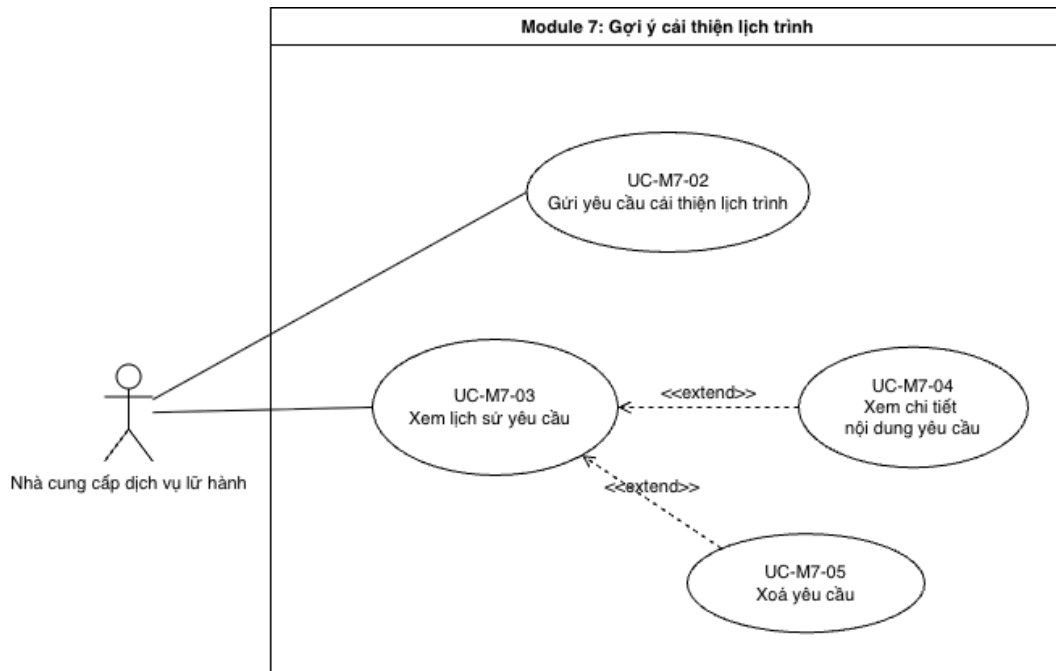
Hình 9: Use case diagram Gợi ý cải thiện lịch trình
