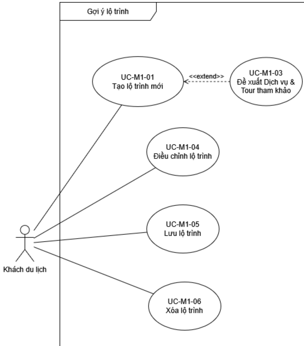
Hình 5: Use case diagram cho Module 1: Gợi ý lộ trình
