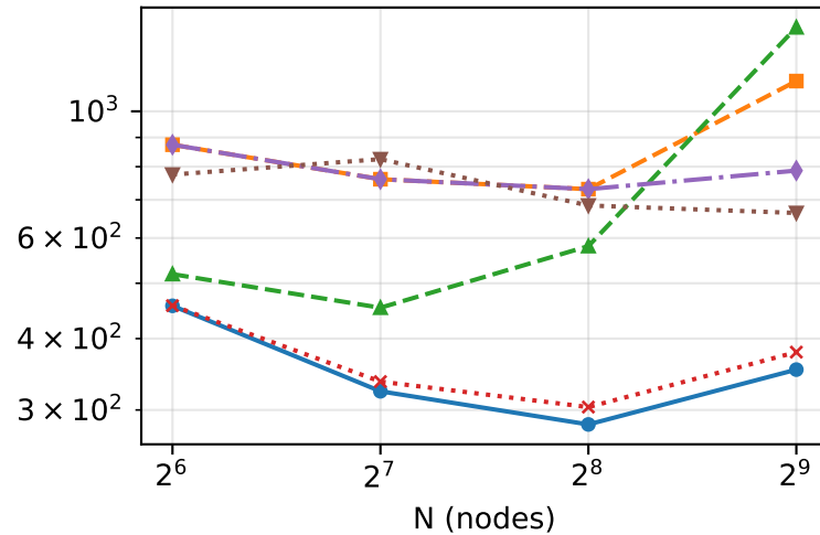
vgg16
