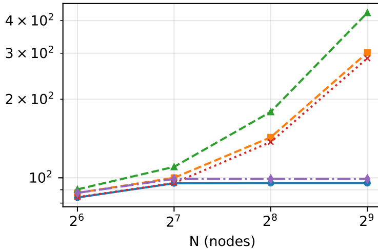
googlenet
