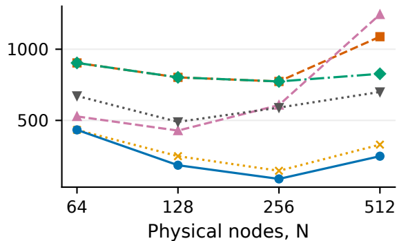
(d) ResNet50
