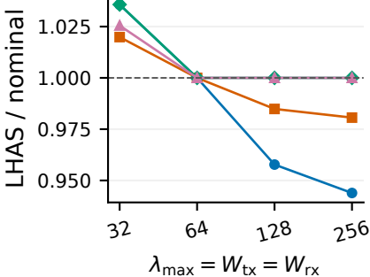
(d) Wavelength / interface budget
