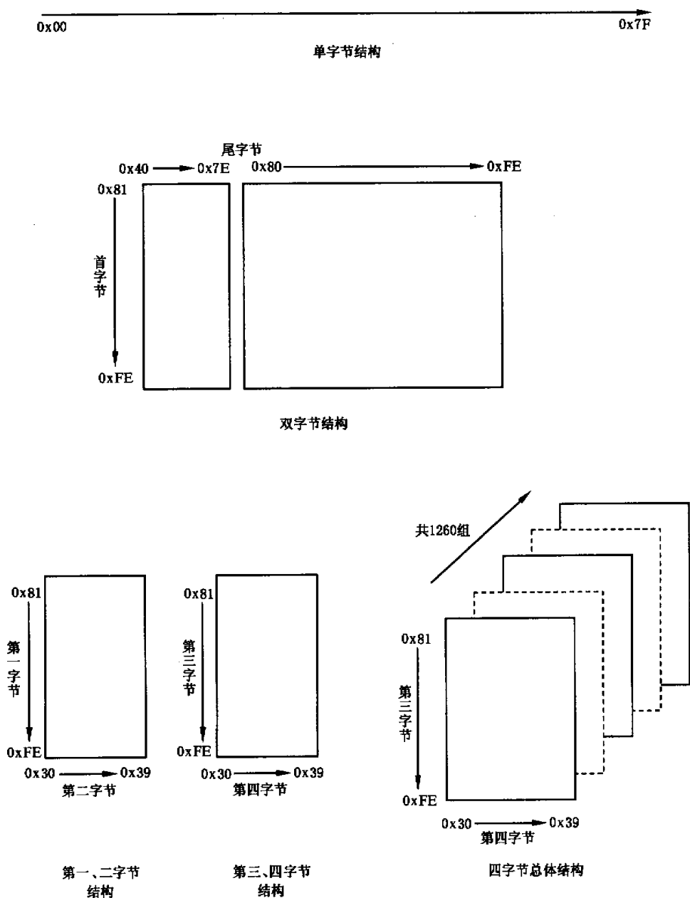
图 1 总体结构图
