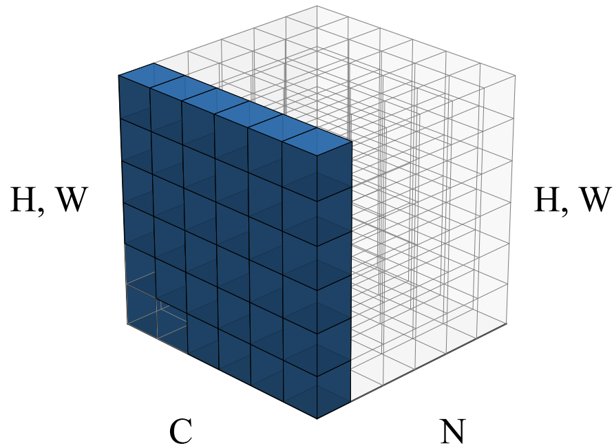
Layer Norm
