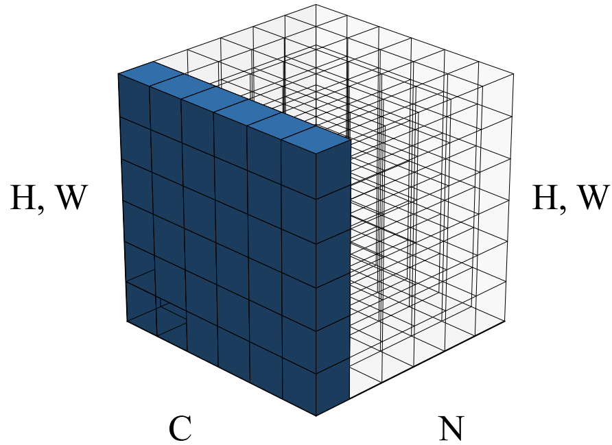
Layer Norm
