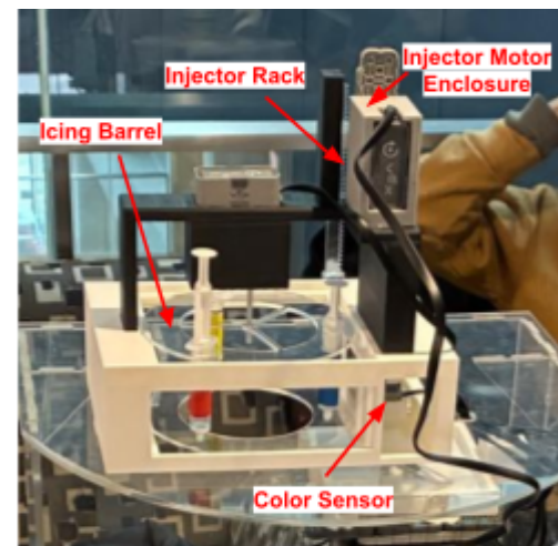
Icing Dispenser
