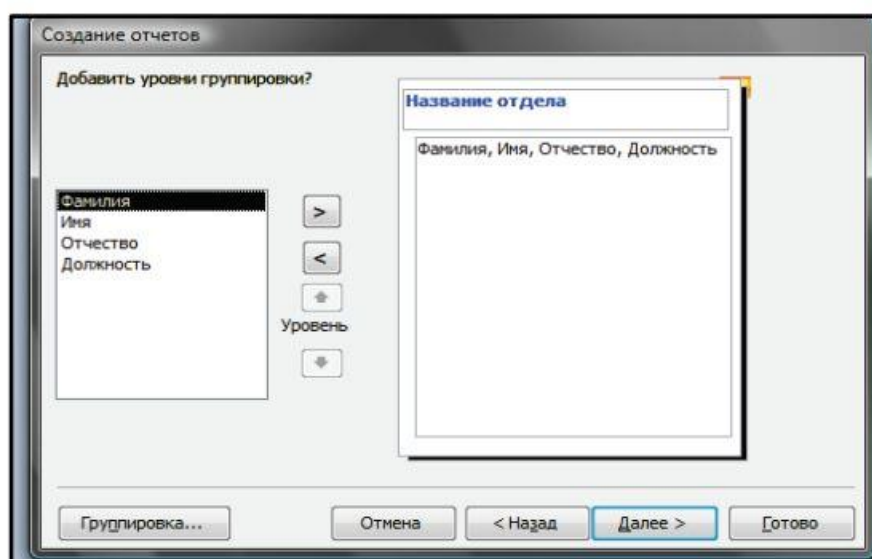
Рис. 29. Группировка данных
