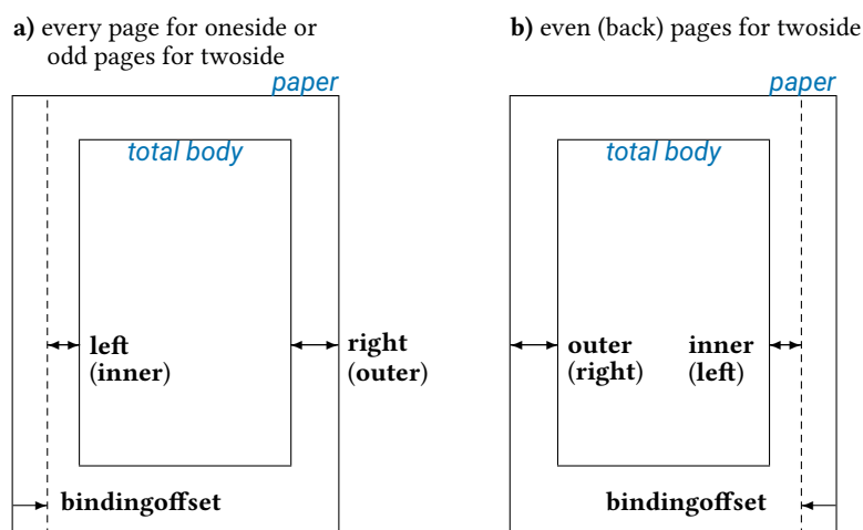
图 6: 参数 bindingoffset 给内页边距加入了确定的长度。注意, twoside 这个参数会交换水平页边距和页边批注还有 bindingoffset 产生的空间 (参见 b), 但是 asymmetric 这个参数不交换页边距和页边批注的位置, 但是会交换 bindingoffset 产生的空间
