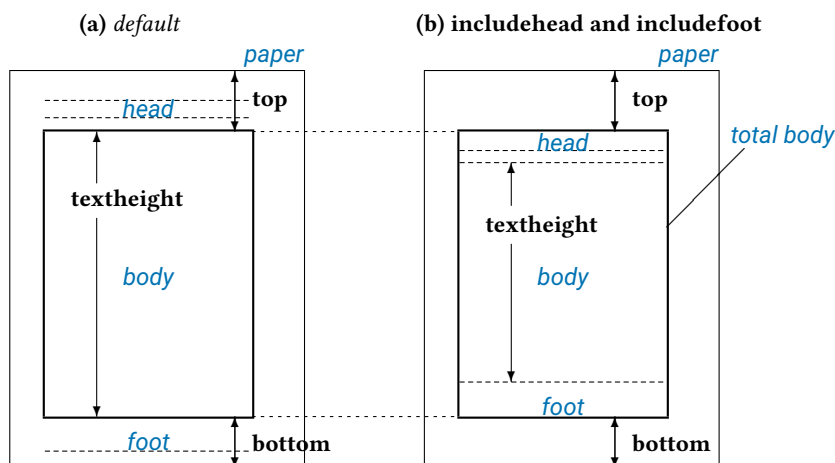
图 2: includehead 和 includefoot 分别将 head 和 foot 包括到了 total body 中。(a) 图表示了 height = textheight (默认值)。(b) 图表示了如果设置了 includehead 和 includefoot , 那么 height = textheight + headheight + headsep + footskip 。显然, 如果定义了 top 和 bottom 参数 includehead 和 includefoot 会导致更短的 textheight 。
