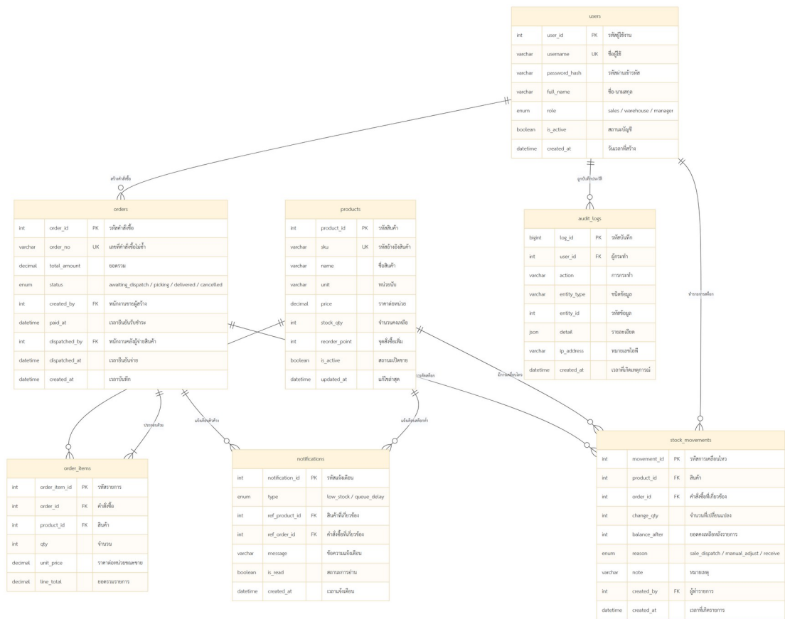
รูปที่ 5 แผนภาพความสัมพันธ์ระหว่างข้อมูล (Entity Relationship Diagram) — จัดตารางตามตารางที่ 3.19 ของปริญญาณิพนธ์
