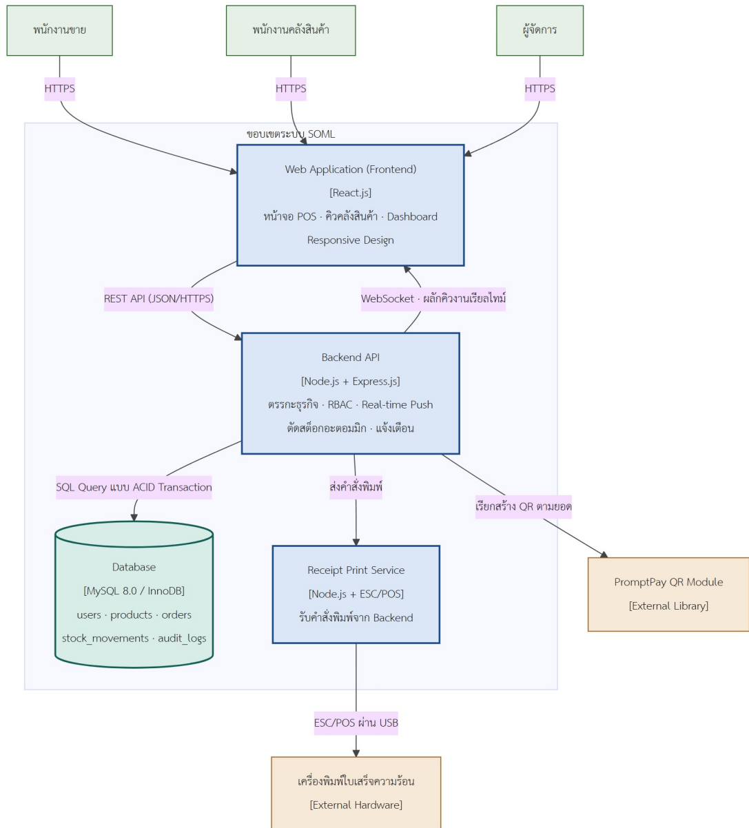
รูปที่ 3 แผนภาพระดับคอนเทนเนอร์ (Container Diagram) — สามชั้นเชิงตรรกะ สี่หน่วยติดตั้ง และสองช่องทางสื่อสารระหว่างหน้าจอกับระบบหลังบ้าน
