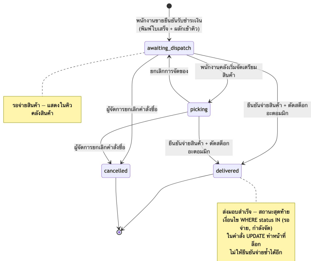
รูปที่ 4 แผนภาพสถานะของคำสั่งซื้อ (Order State Diagram) — สถานะส่งมอบสำเร็จเข้าถึงได้เฉพาะผ่านธุรกรรมตัดสต็อก และย้อนกลับไม่ได้
