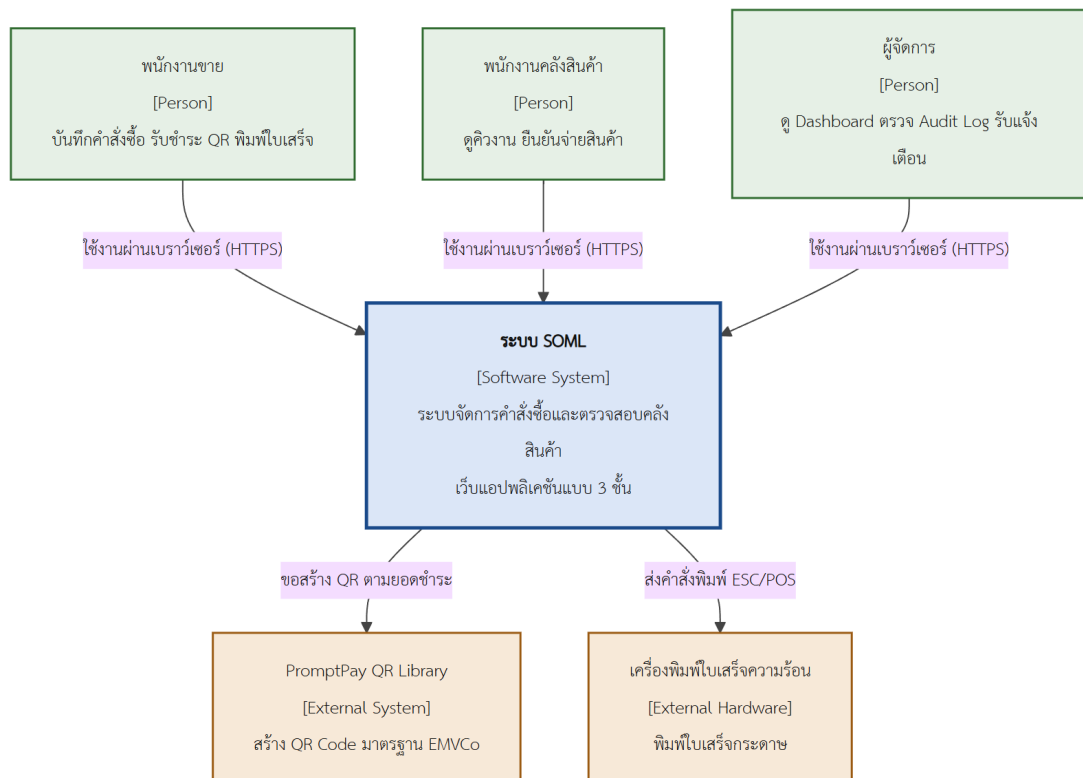
รูปที่ 1 แผนภาพบริบทของระบบ (Context Diagram) — ผู้ใช้สามบทบาท ระบบ SOML และองค์ประกอบภายนอกสองรายการ
