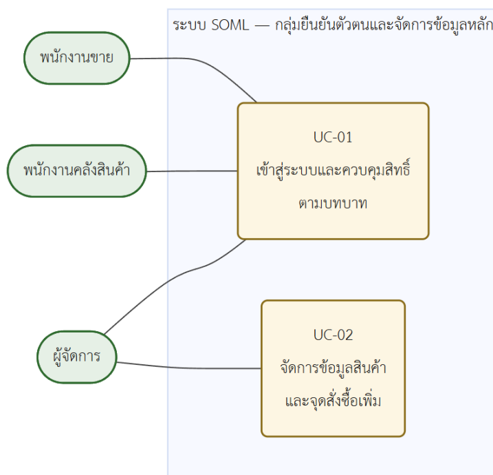
รูปที่ 3.2 แผนภาพกรณีการใช้งานกลุ่มการเข้าสู่ระบบและควบคุมสิทธิ์
