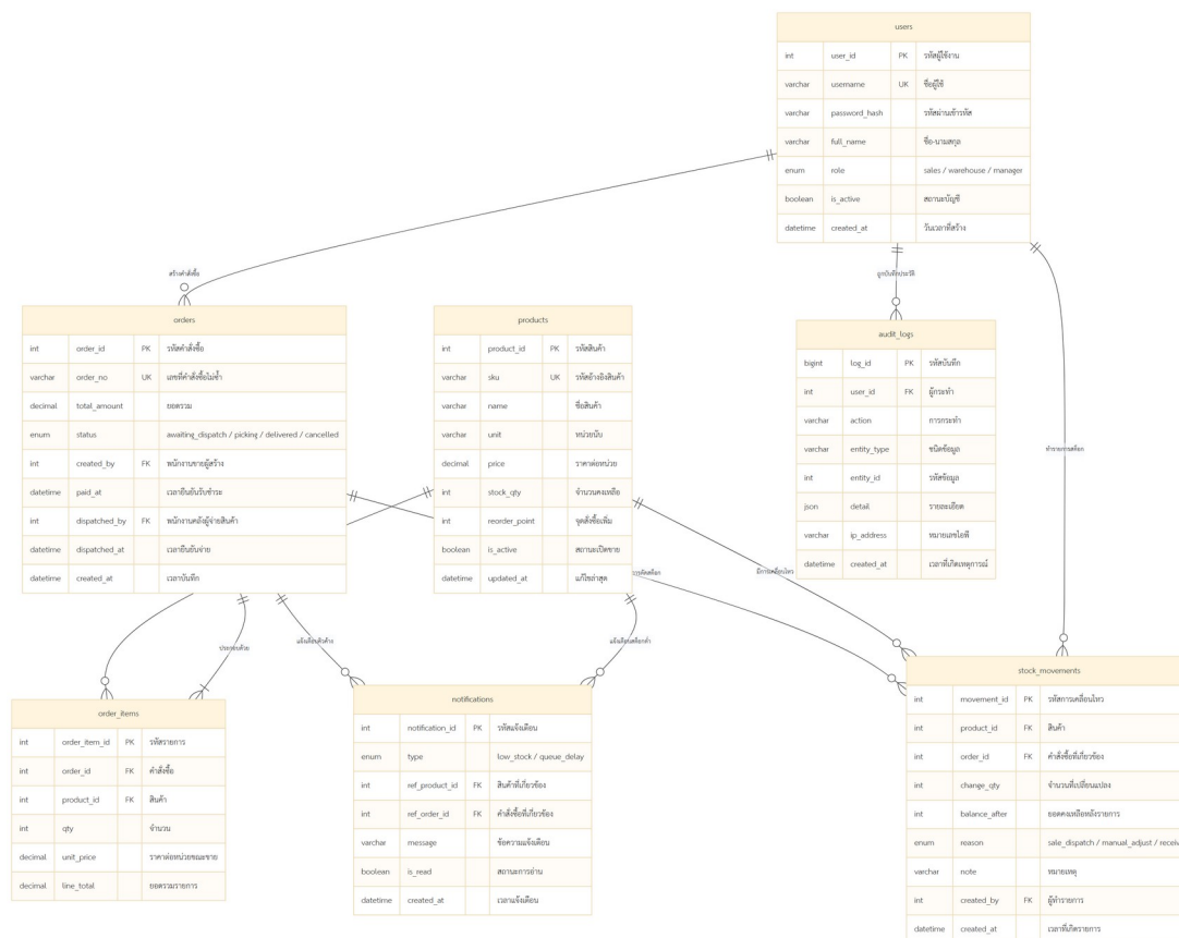
รูปที่ 3.9 แผนภาพความสัมพันธ์ระหว่างข้อมูล (Entity Relationship Diagram)
