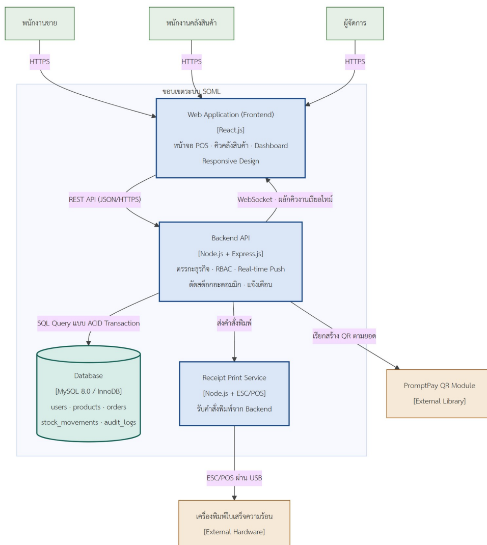
รูปที่ 3.7 แผนภาพระดับคอนเทนเนอร์ของระบบ (C2: Container Diagram)
