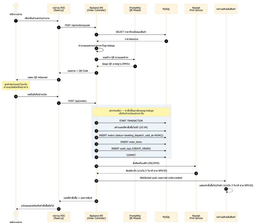
รูปที่ 3.10 แผนภาพลำดับของการสร้างคำสั่งซื้อและออกใบเสร็จ (Sequence Diagram: UC-03)
