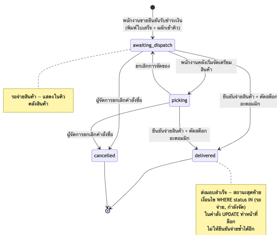
รูปที่ 3.13 แผนภาพสถานะของคำสั่งซื้อ (Order State Diagram)
