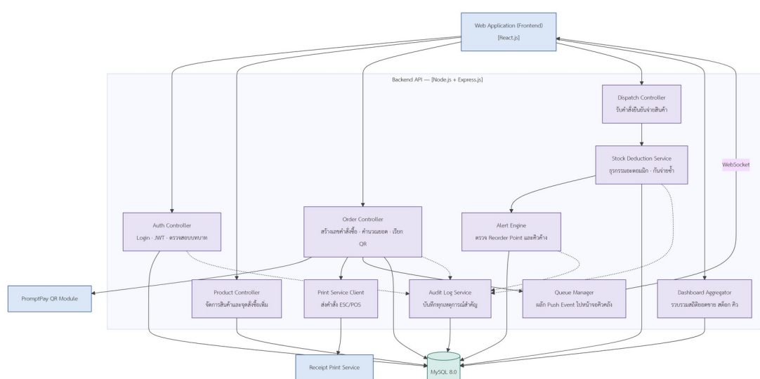
รูปที่ 3.8 แผนภาพส่วนประกอบภายในระบบหลังบ้าน (C3: Component Diagram)
