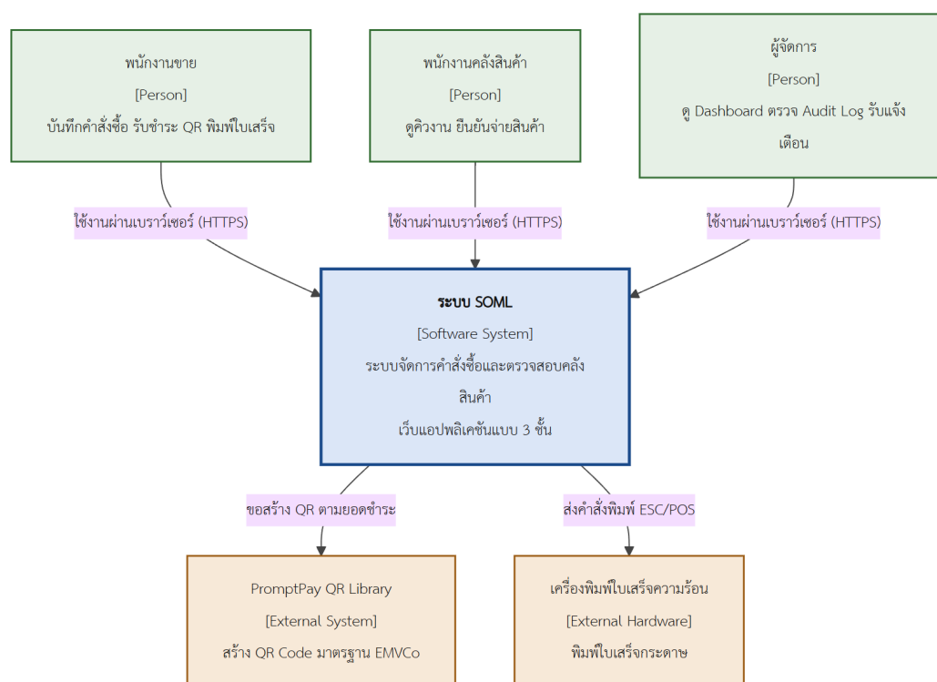
รูปที่ 3.6 แผนภาพบริบทของระบบ (C1: System Context Diagram)
