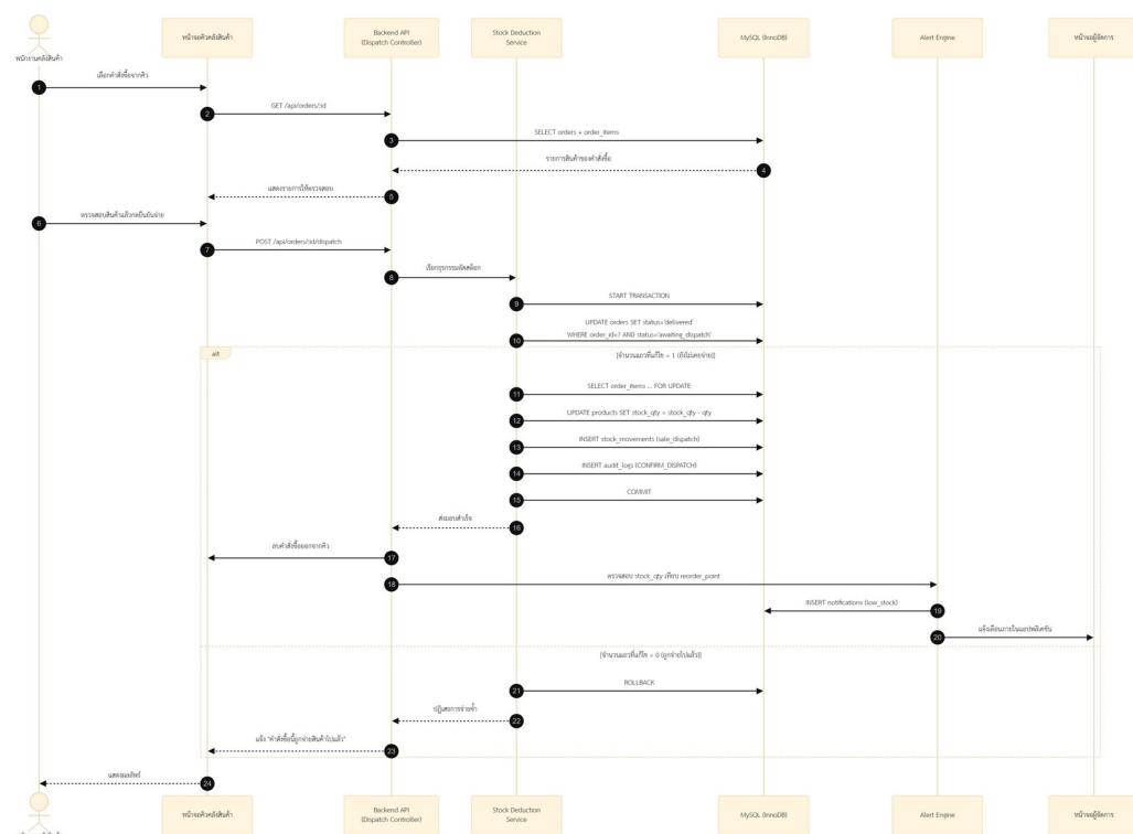
รูปที่ 3.11 แผนภาพลำดับของการยืนยันจ่ายสินค้าและตัดสต็อก (Sequence Diagram: UC-07)
