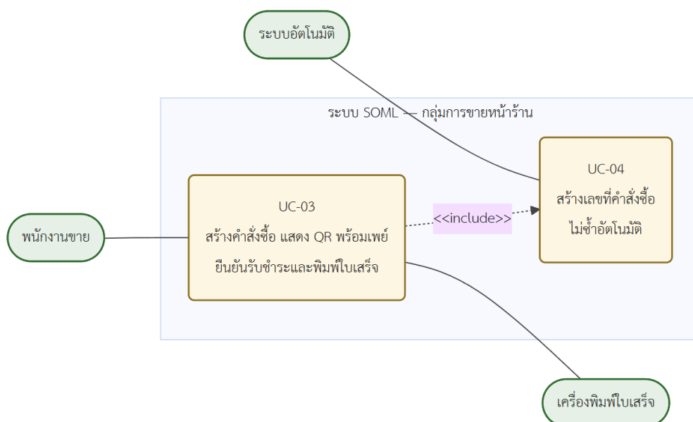
รูปที่ 3.3 แผนภาพกรณีการใช้งานของพนักงานขาย
