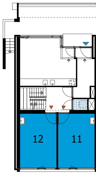
2e verdieping 2nd floor
