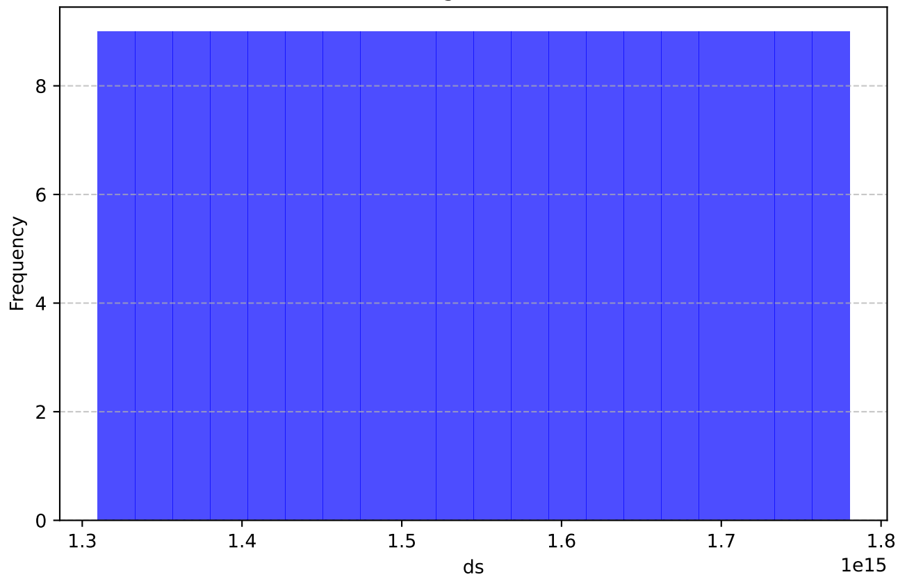
Histogram of ds
