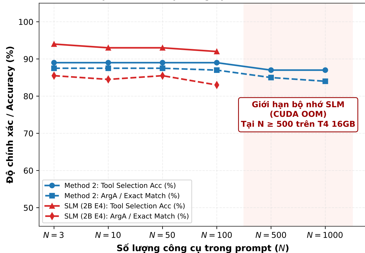
(a) Độ chính xác chọn công cụ & trích xuất tham số
