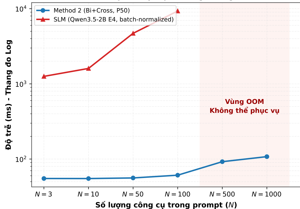
(b) Độ trễ suy luận (Thang đo Log)
