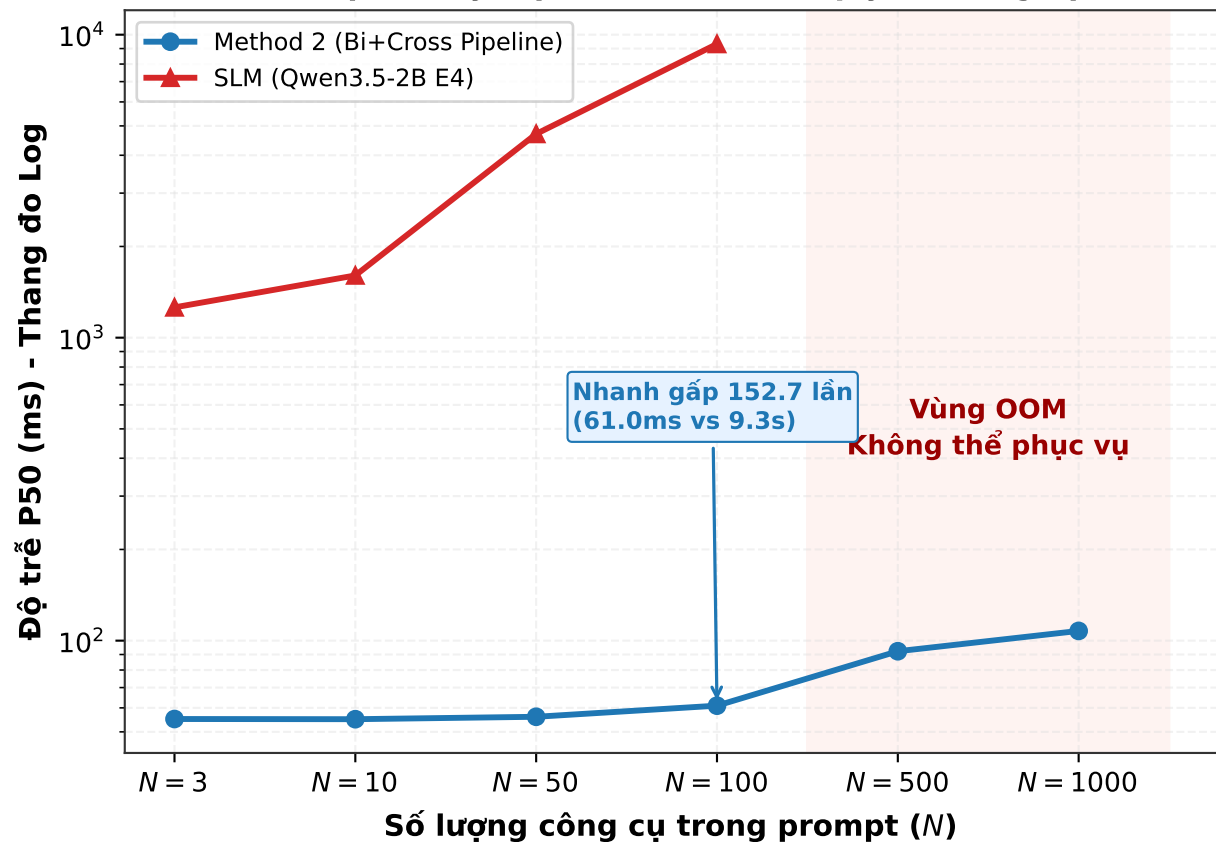
(b) Độ trễ suy luận P50 (ms) theo quy mô công cụ
