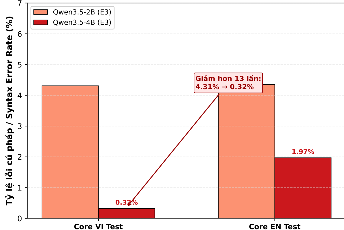
(b) Triệt tiêu lỗi cú pháp JSON (Syntax Error)
