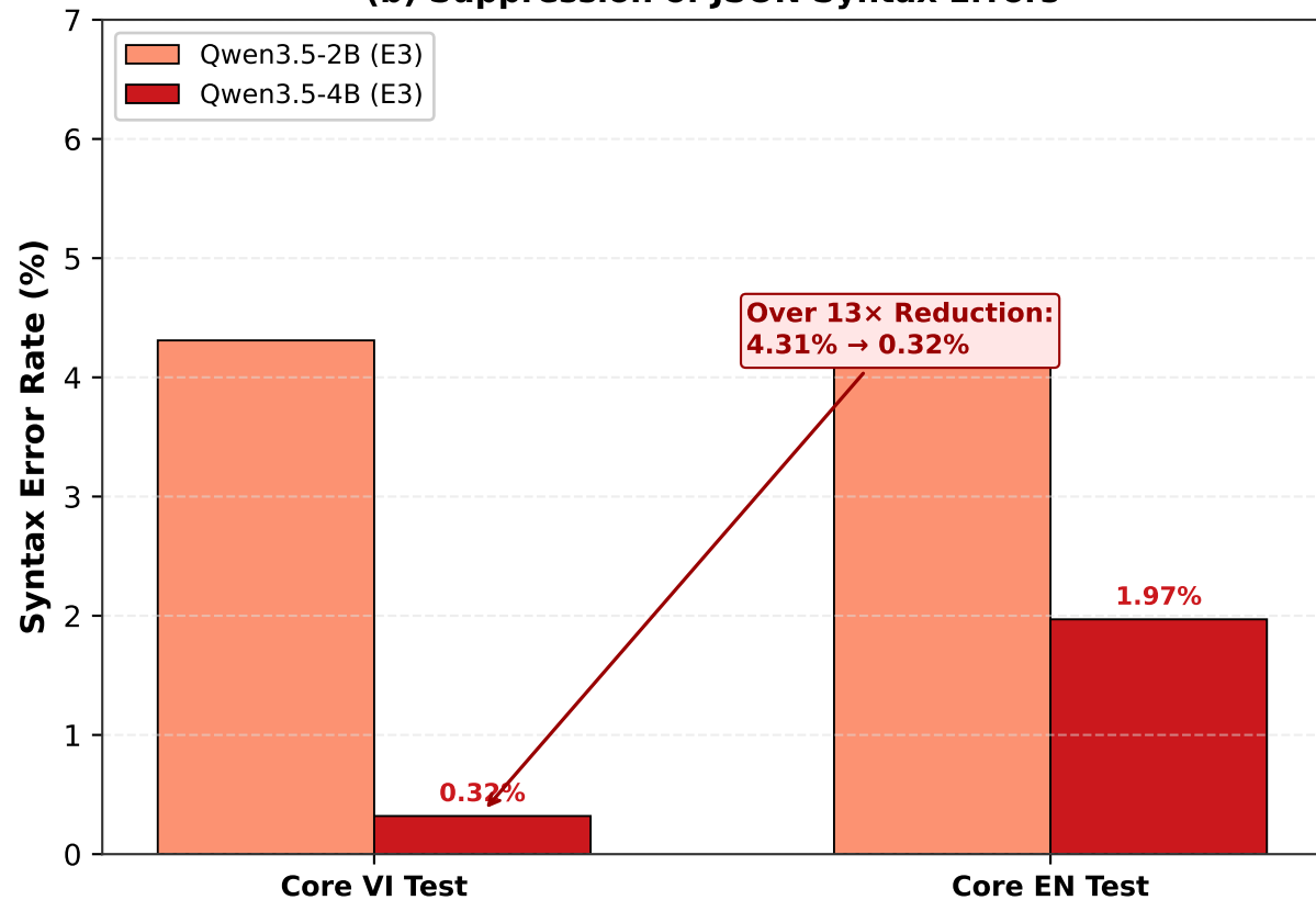
(b) Suppression of JSON Syntax Errors
