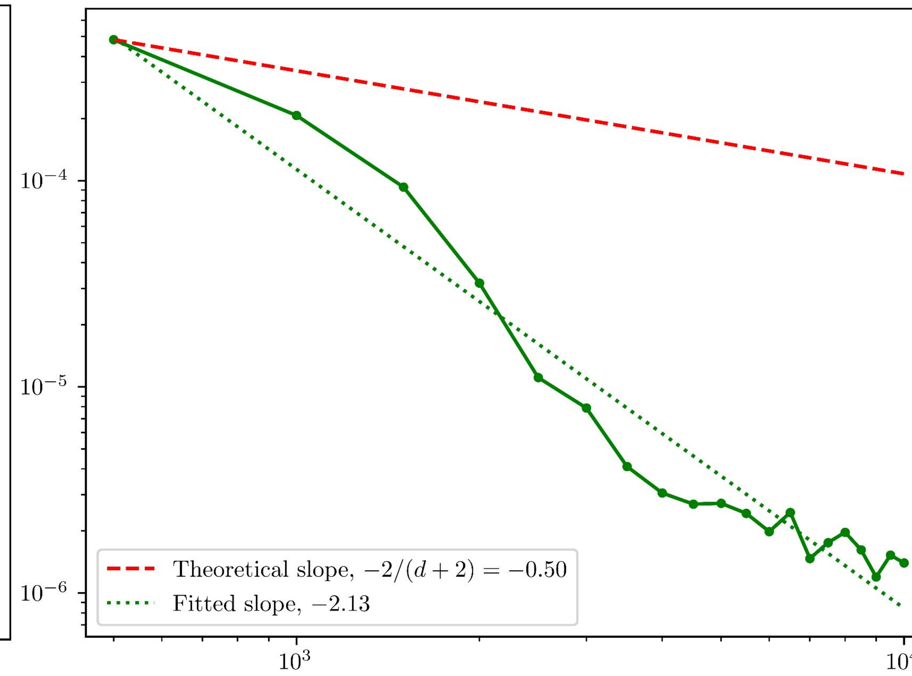
Circle
