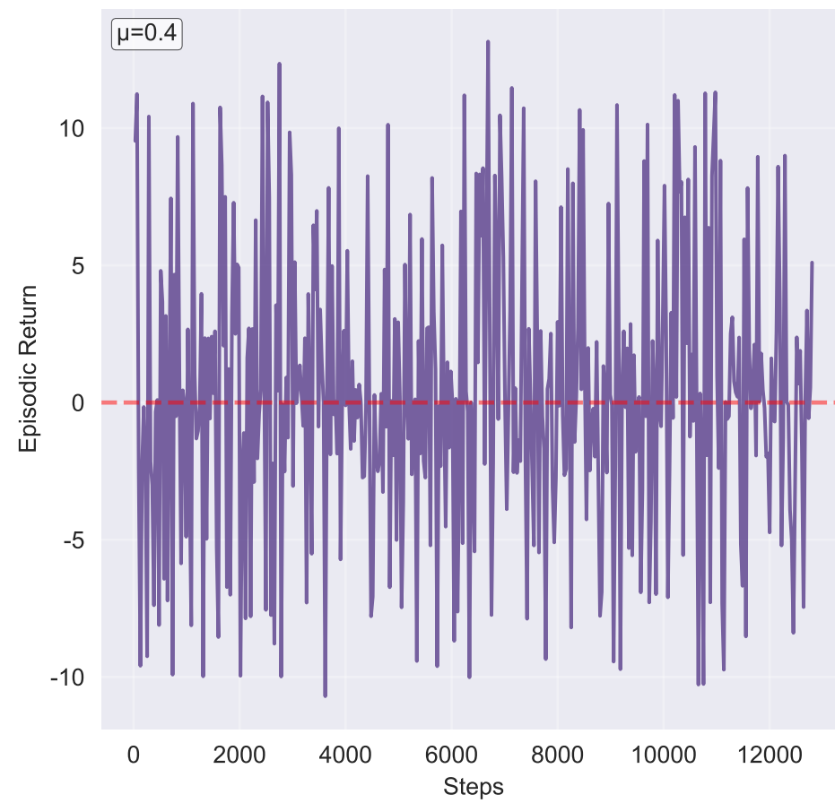
Softmax
