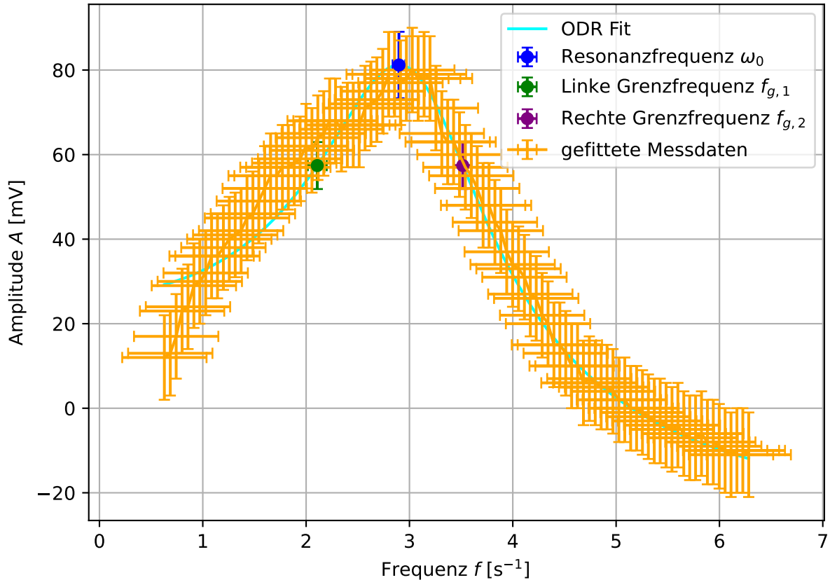
Messung 7 bei Stromstärke 0.75 A
