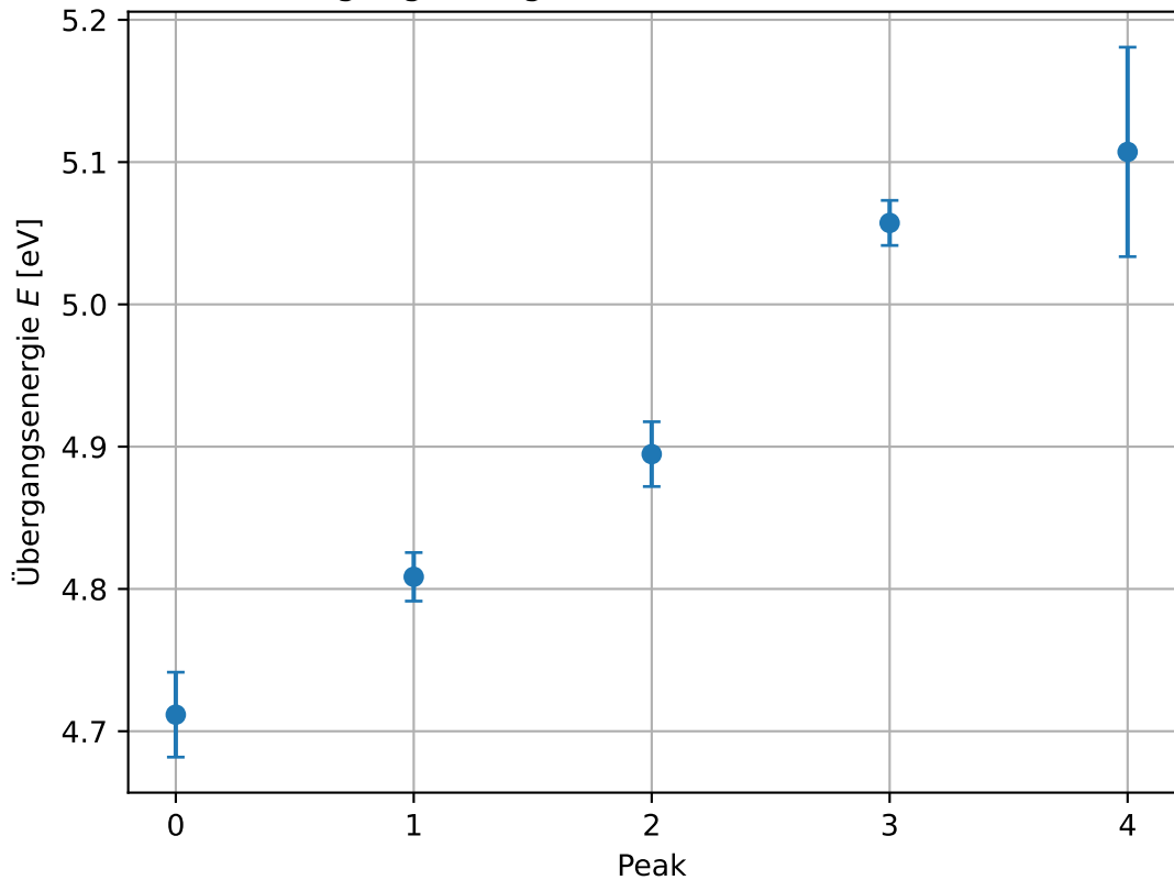
Übergangsenergie für unterschiedliche Peaks
