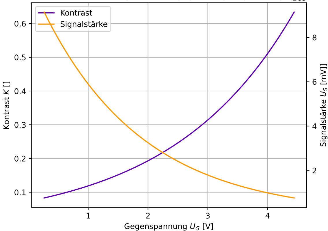
Kontrast und Signalstärke gegen Gegenspannung 1e3
