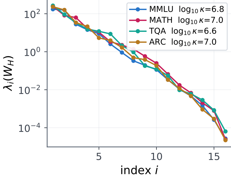
(d) Gemma-2-9B
