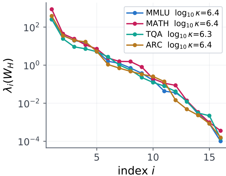
(d) Gemma-2-9B
