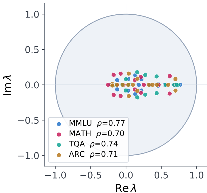
(d) Gemma-2-9B
