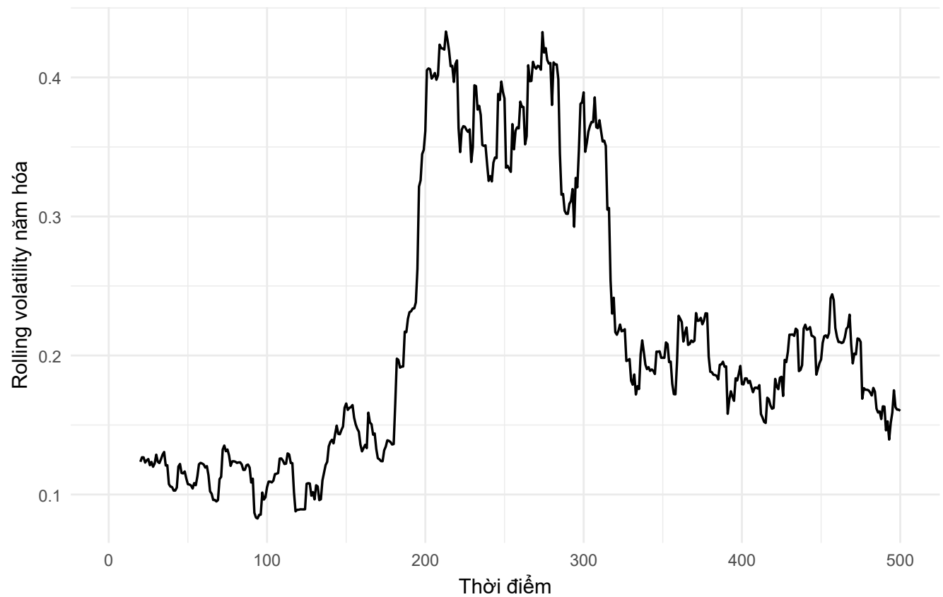
Rolling volatility thay đổi theo thời gian
